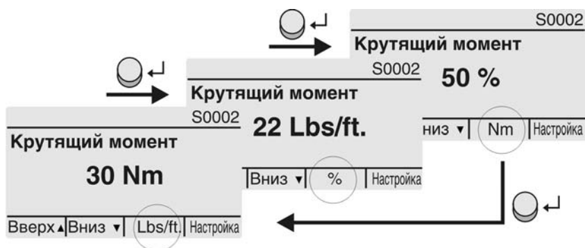
рис. 46: Единицы измерения крутящего момента
