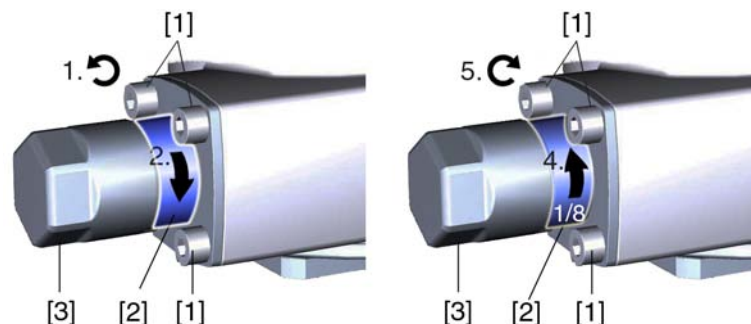
рис. 61: концевой упор
