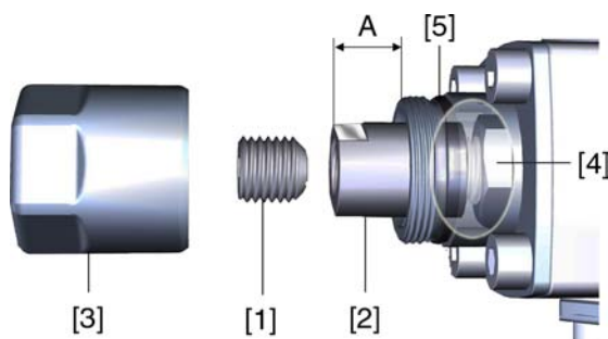
рис. 64: концевой упор
