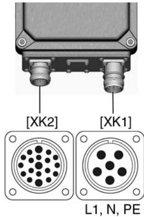
рис. 7: Распределение клемм
