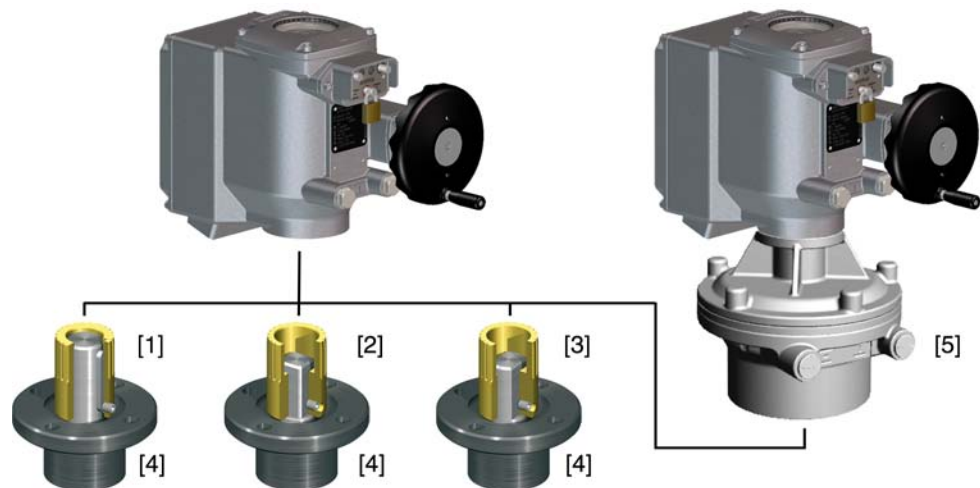
рис. 4: Варианты втулок
