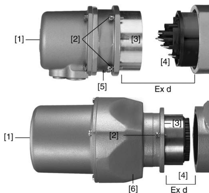
рис. 45: сверху: КР/КРН, внизу: KES
