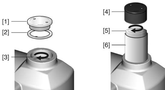
рис. 36: Пустотелый вал/шток
