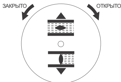
рис. М-1: Диск указателя положения
