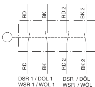
II последовательный переключатель
