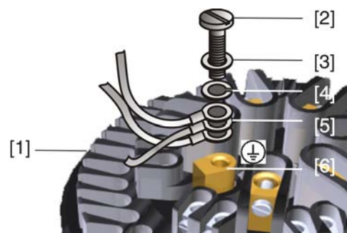
рис. 18: Заземляющий контакт
