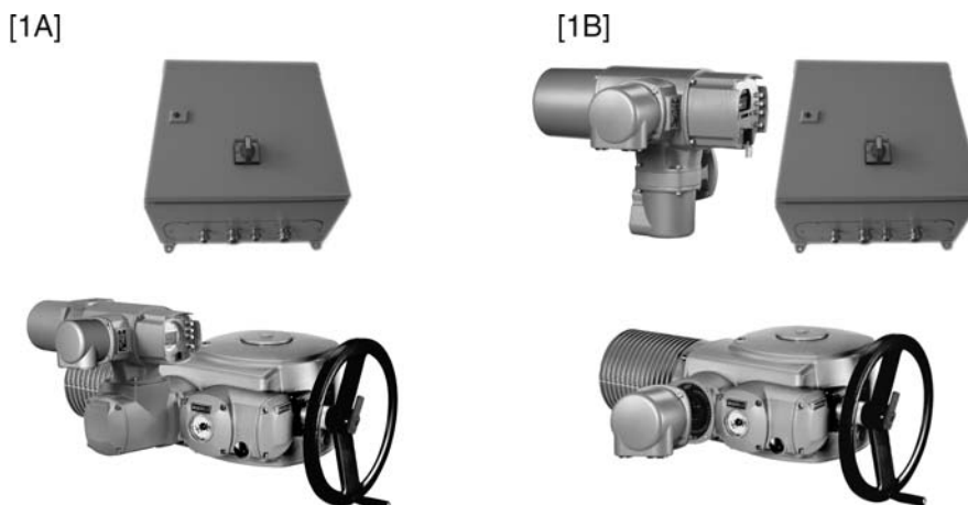
рис. 14: Монтаж блока управления
