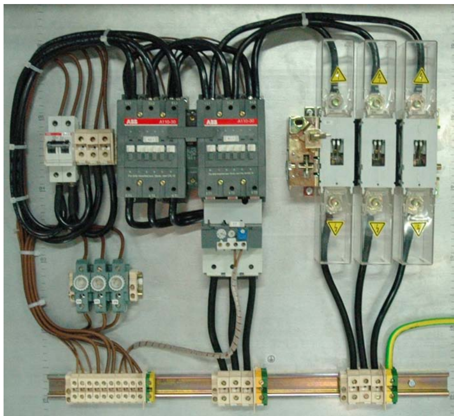
рис. 55: Распределительная коробка
