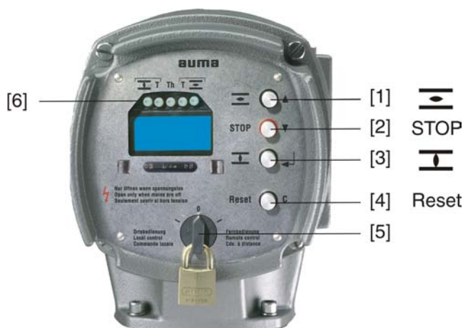
рис. 27: Панель местного управления
