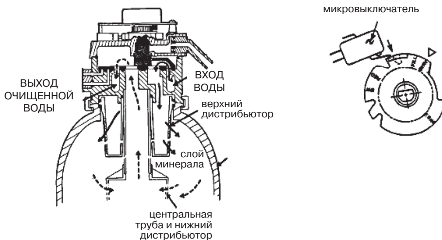
Рис. 10. Рабочий цикл
