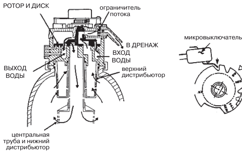
Рис. 11. Обратная промывка
