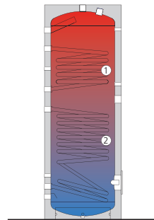
1. Scambiatore superiore per integrazione al sanitario. (generatore) 2. Scambiatore solare termico
