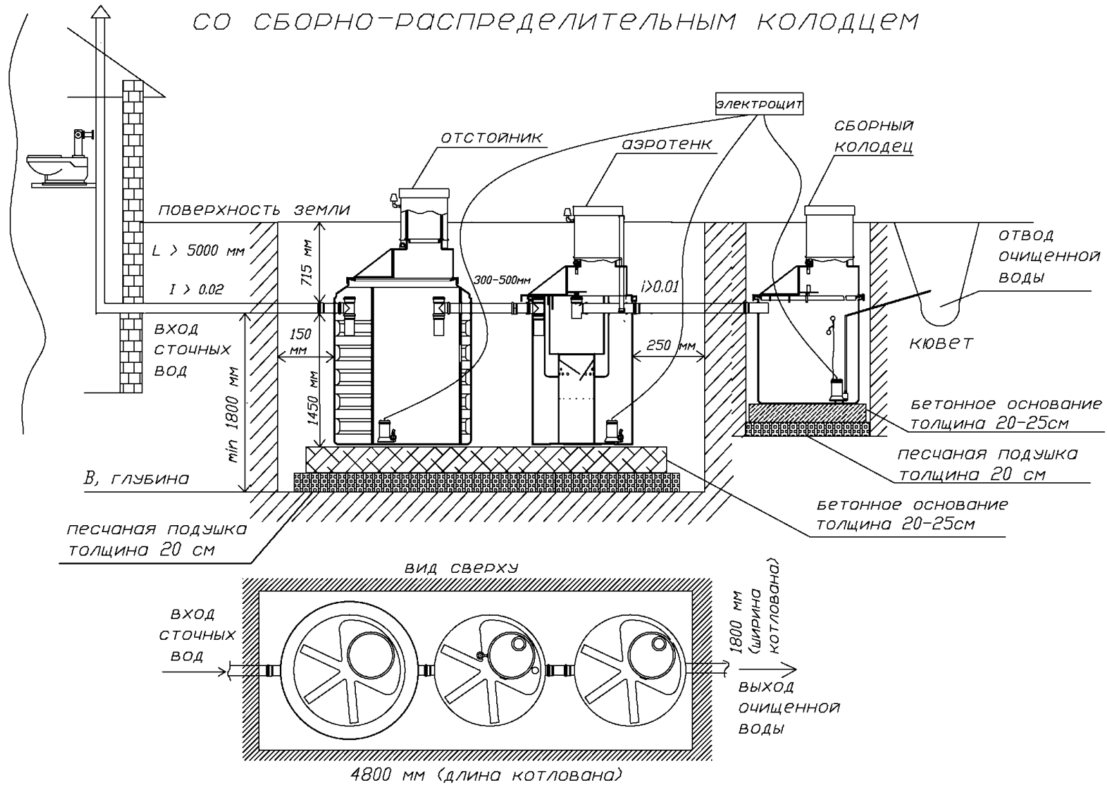
3.2 Монтажная схема ЛОС 15 со сборным колодцем (пльвун)
