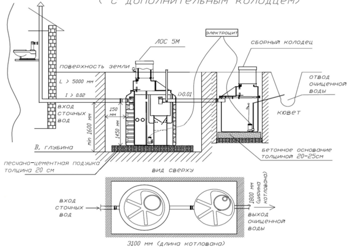
рис. 4.1. Монтажная схема ЛОС 5М со сборным колодцем (песок, суглинок, глина)
