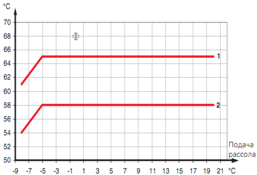
1. Выход конденсатора 2. Вход конденсатора
