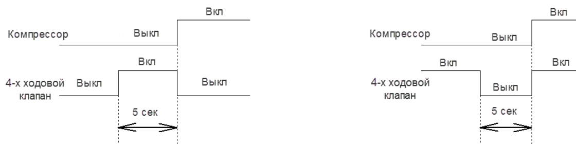
Включение/выключение 4х ходового клапана в режиме нагрева
