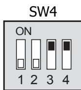
Режим отопления и охлаждения и горячее водоснабжение (ГВС)
