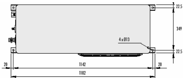
ВИД СВЕРХУ
