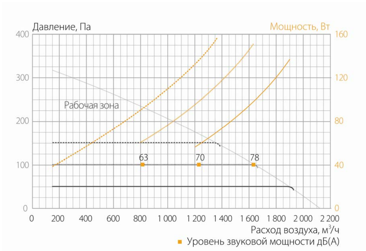
Вентилятор VCZ1086RU
