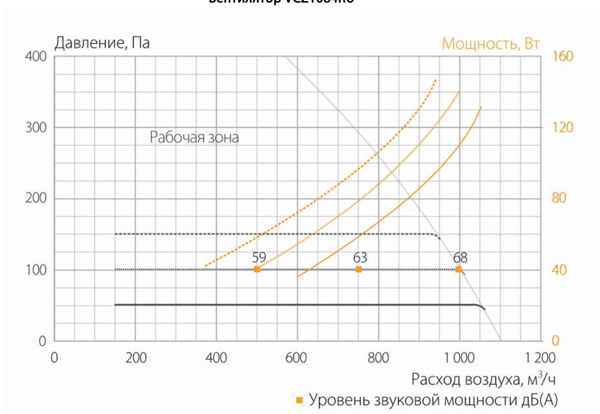
Вентилятор VCZ1085RU
