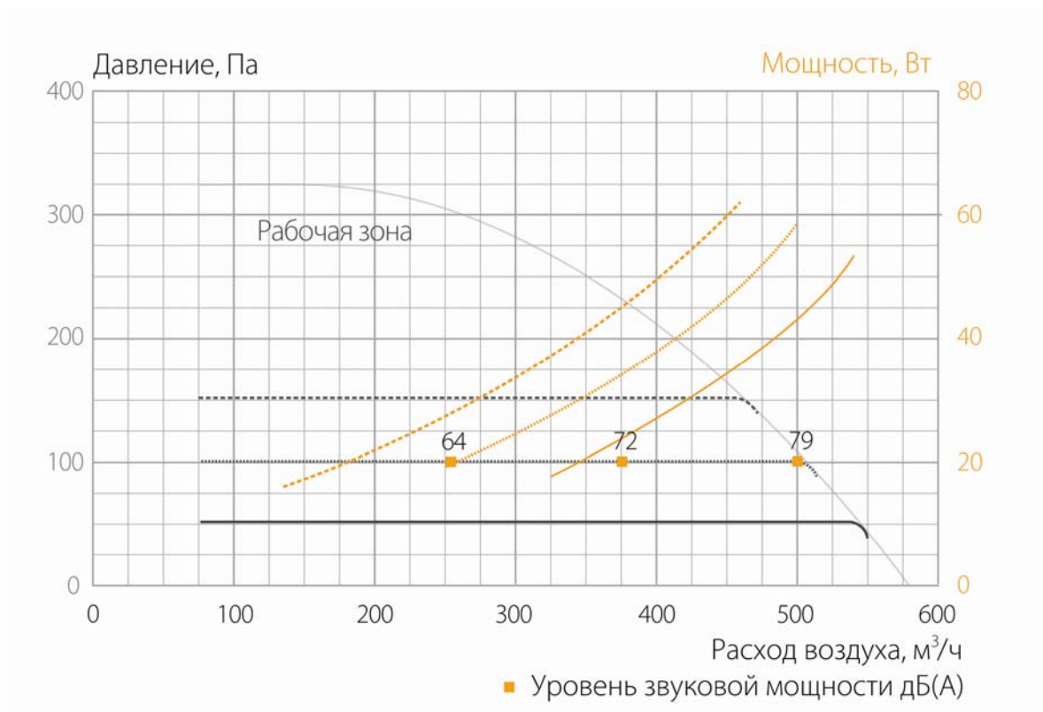
Вентилятор VCZ1084RU
