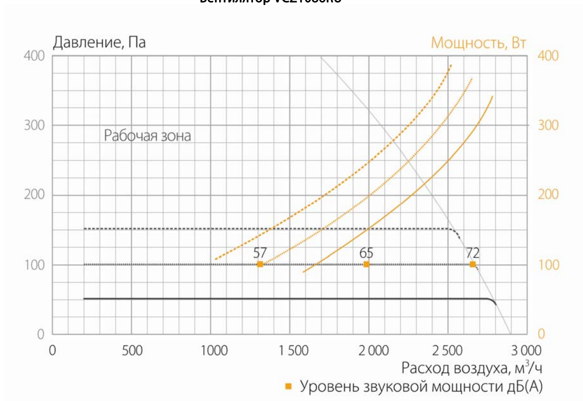
Вентилятор VCZ1087RU
