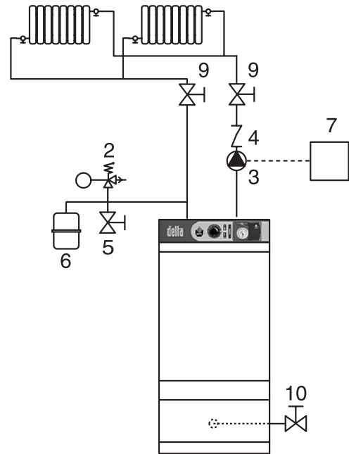
Рис. 2: Гидравлическая схема с управлением циркуляционным насосом от комнатного термостата.
