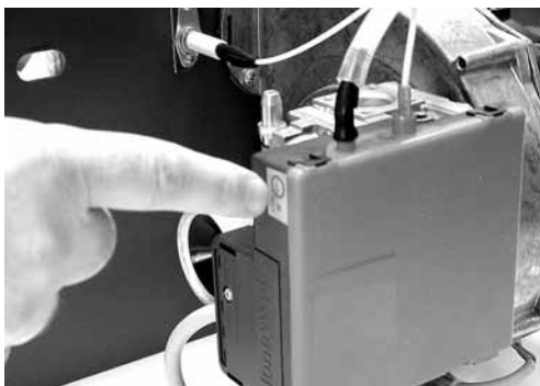
Рис. 25: Кнопка перезапуска горелки
