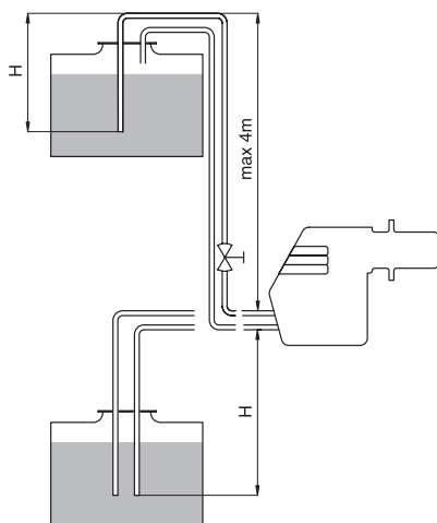
Рис. 8b: Питание топливом с обратной магистралью при высоко или низко расположенном баке
