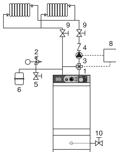
Рис. 3: Гидравлическая схема с 3-х ходовым смесителем с электроприводом.
