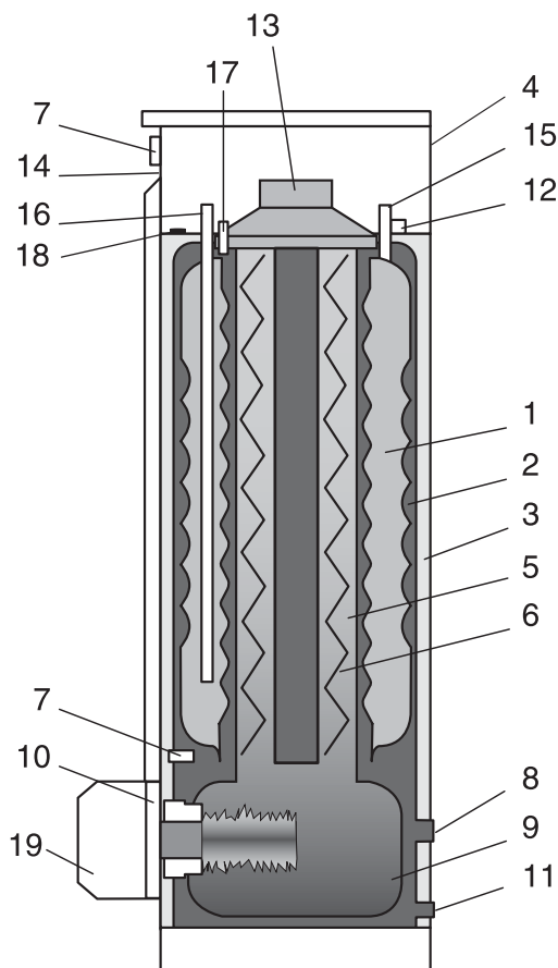
Рис. 16: Устройство котла
