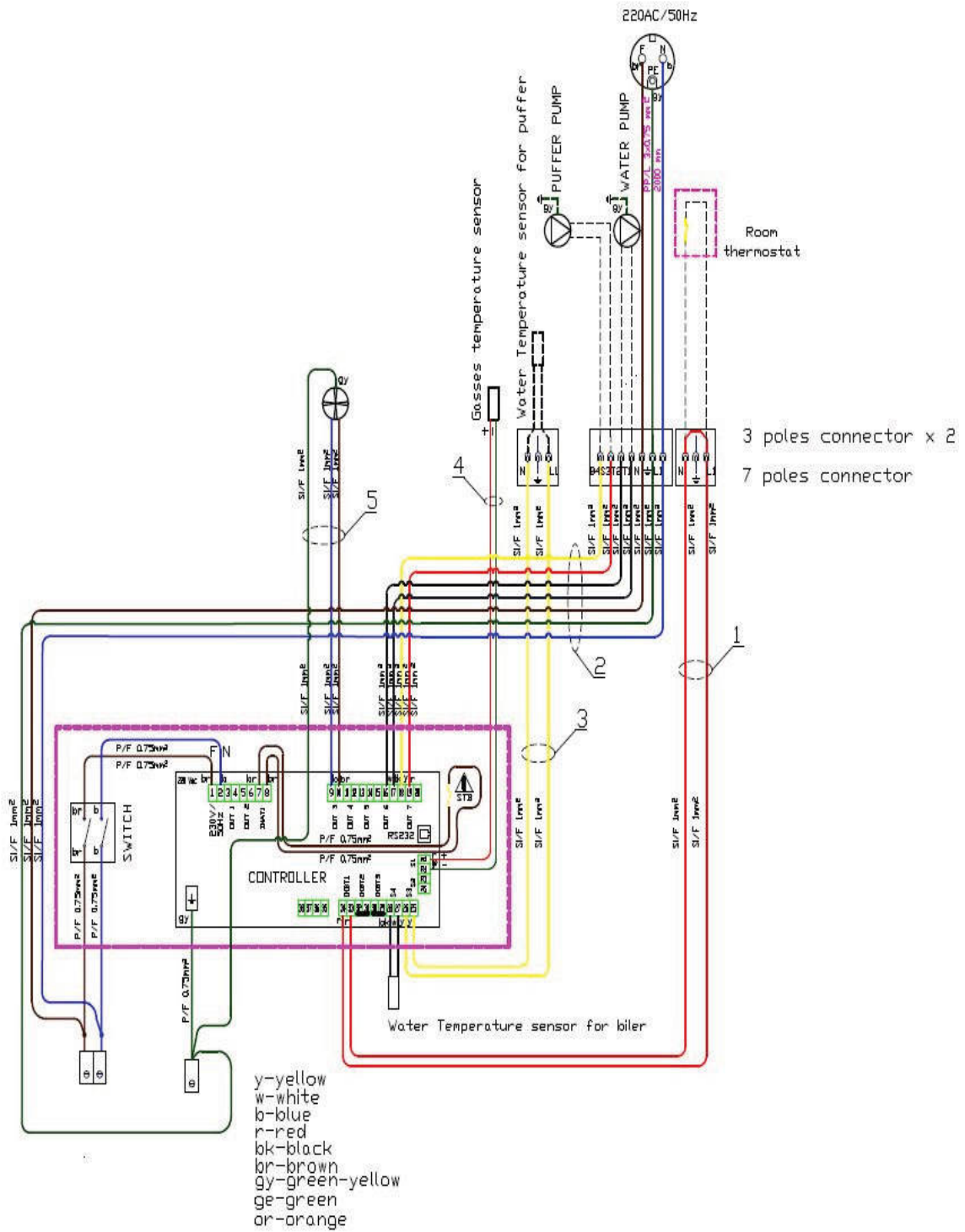
Электрические подключения
