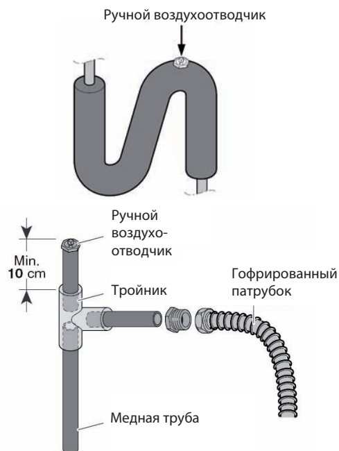
Рис. 6. Установка воздухоотводчиков
