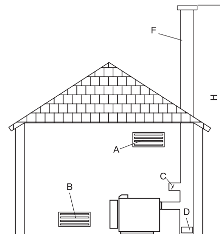
Рис. 1: Присоединение котла к дымоходу
