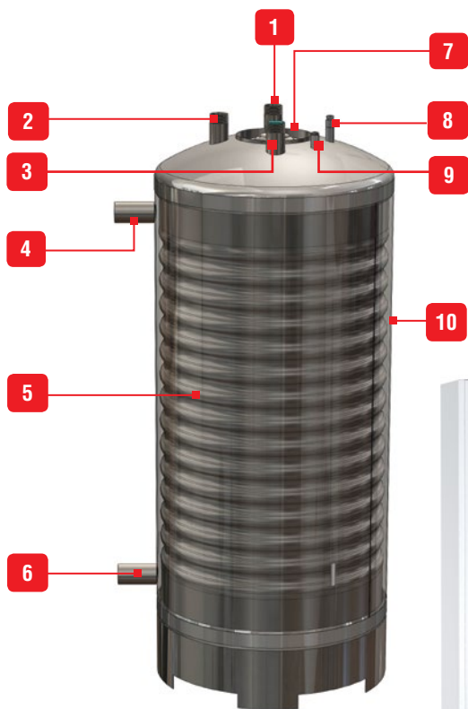
Водонагреватель показан без теплоизоляции
