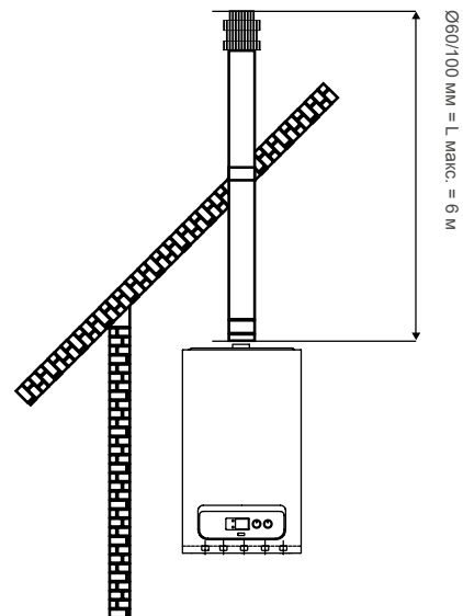
Рисунок 18 Вертикальный монтаж дымохода
