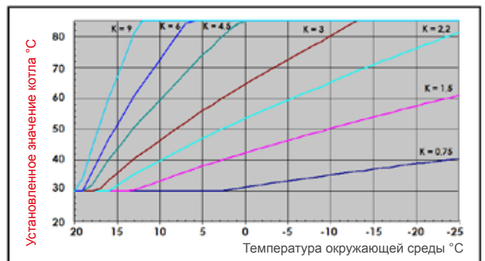
Рисунок 33. Кривая эксплуатации внешнего датчика температуры
