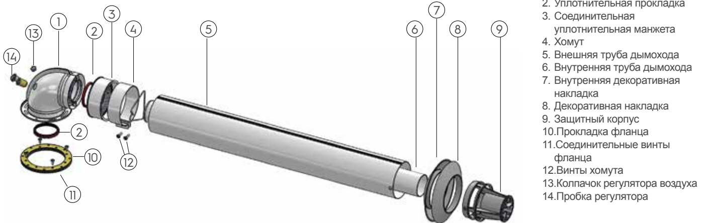
Рисунок 11. Дымоход котла
