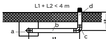
Рисунок 16 II. Монтаж дымохода с двумя угловыми отводами 90°.
