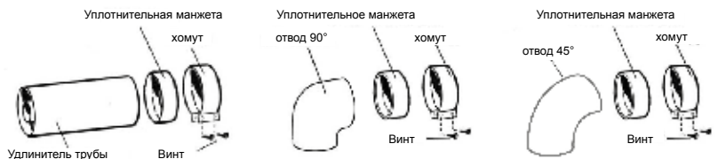
Рисунок 13. Монтаж элементов дымохода
