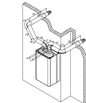
Рисунок 20 Монтаж герметичного дымохода
