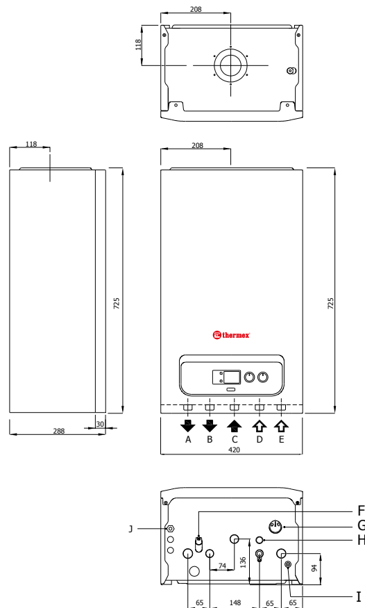
Рисунок 6. Размеры и подключения котла Xantus
