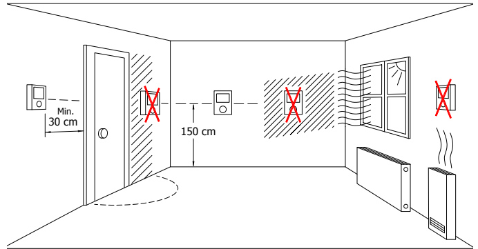
Рисунок 31. Положение термостата
