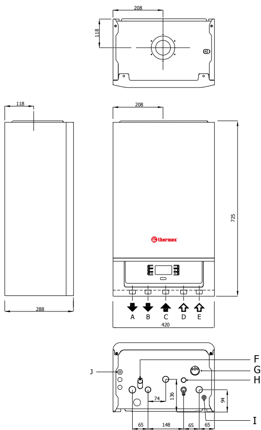
Рисунок 7. Размеры и подключения котла XantusPlus
