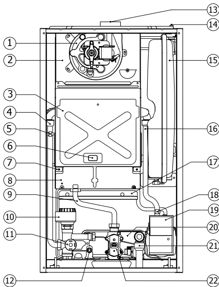
Рисунок 25. Компоненты котла
