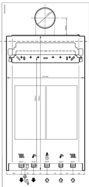
Рисунок 1. Шаблон/схема монтажа
