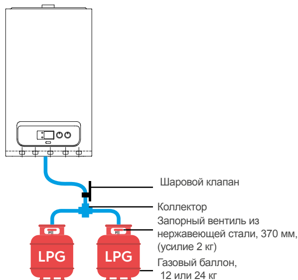
Рисунок 8. Газовое подключение котла
