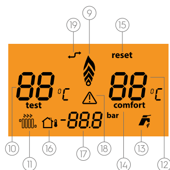
Рисунок 29. Экран автоматической панели управления XantusPlus
