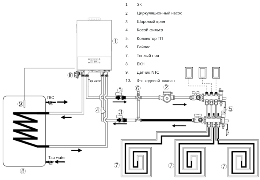
Рис. 16 Схема подключения «ЭЖ + БКН + теплый пол»
