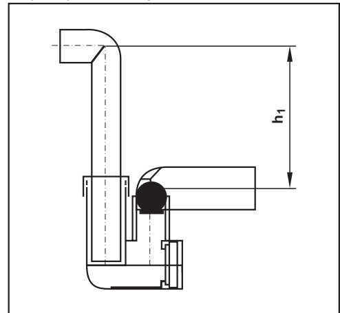
Шарообразный сифон
