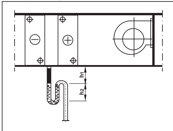
Стандартный сифон
