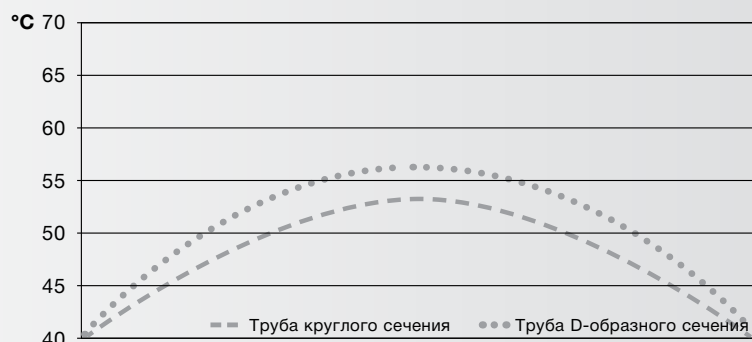
Труба круглого сечения: максимальное/среднее значение = 53,2 °C/47,5 °C Труба D-образного сечения: максимальное/среднее значение = 55,8 °C/49,5 °C
