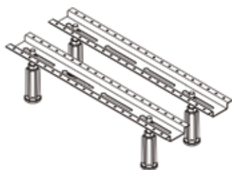
Ножки для ванн, Mauersberger, для ванн до 1800*800 мм, 4 регулируемые по высоте, передвижные ножки, диапазон для регулировки высоты 125–195 мм
