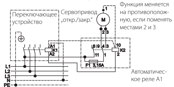
Схема соединений в сочетании с устройством LH
