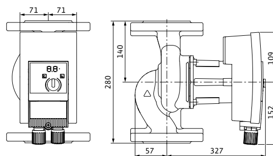
Yonos MAXO 65/0,5-9
