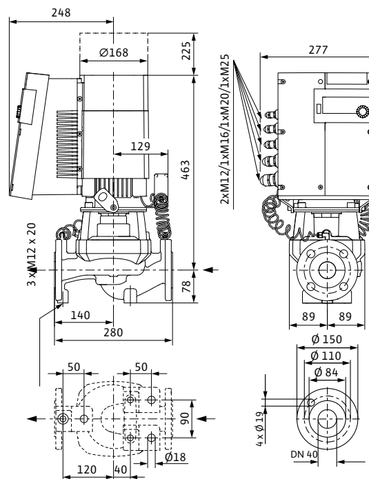
Stratos GIGA 40/1-32/2,3
