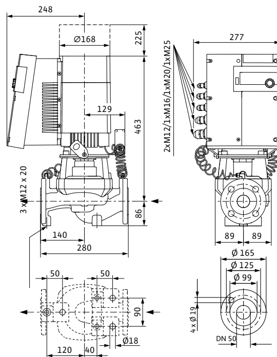
Stratos GIGA 50/1-50/4,5
