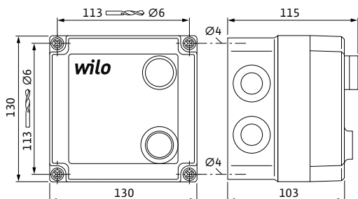
Габаритный чертеж SK 622N
