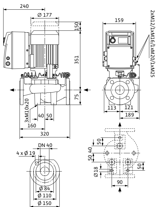
Wilo-VeroLine-IP-E 40/120-1,5/2
