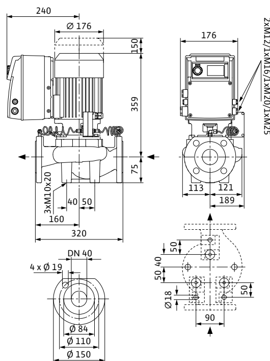
Wilo-VeroLine-IP-E 40/130-2,2/2
