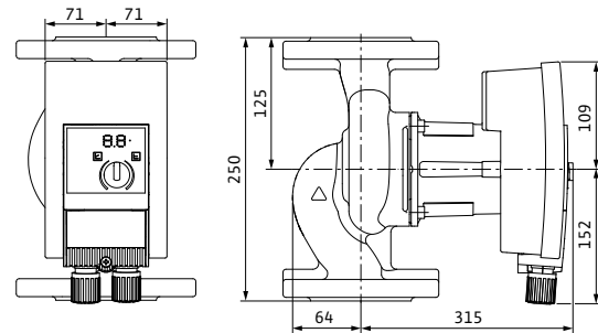
Yonos MAXO 40/0,5-12
