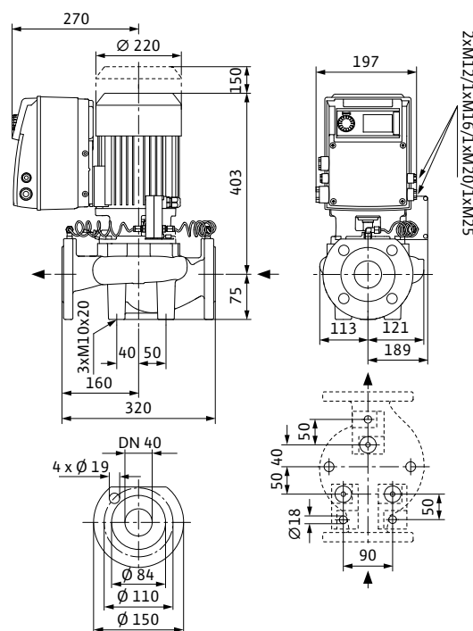
ВeroLine-IP-E 40/160-4/2
