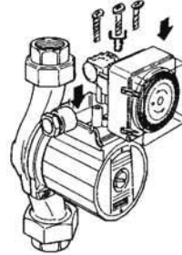
Рис.: Монтаж временного модуля S1R-h
