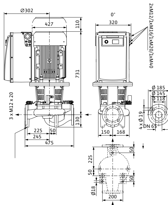
CronoLine-IL-E 65/220-22/2
