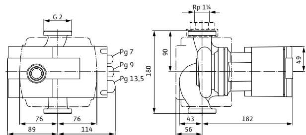
Stratos 30/1-10
