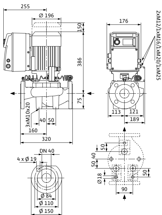
ВeroLine-IP-E 40/150-3/2
