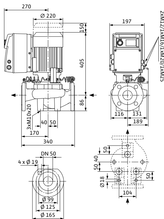
VerоLine-IP-E 50/150-4/2
