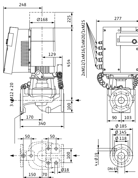
Stratos GIGA 65/1-21/2,3
