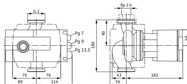
Stratos 30/1-8
