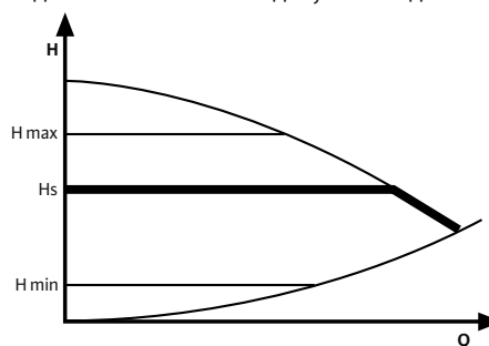
Рис.: Способ регулирования \Delta p-s
