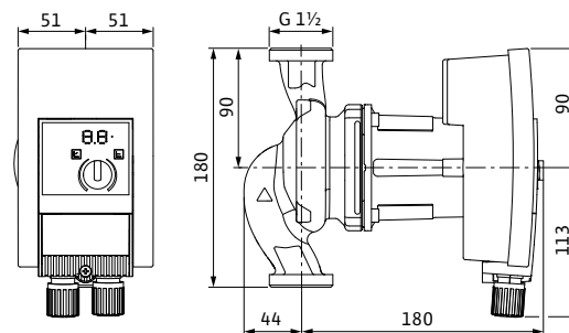
Yonos MAXO 25/0,5-10
