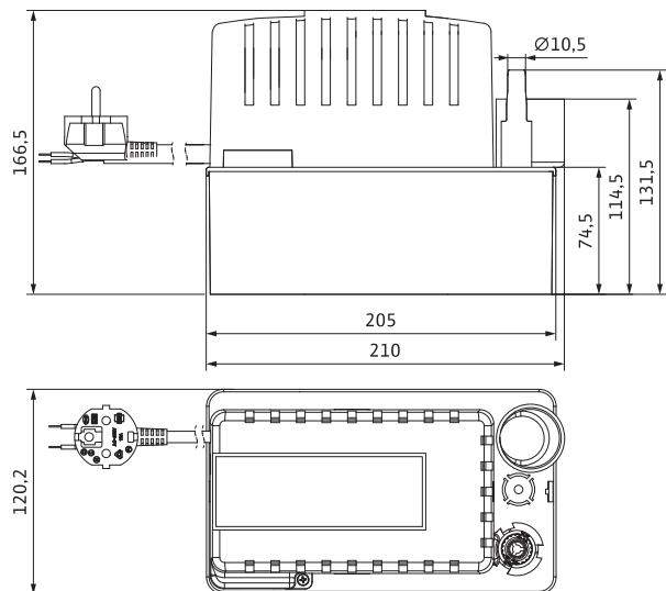
Wilo-DrainLift Con
