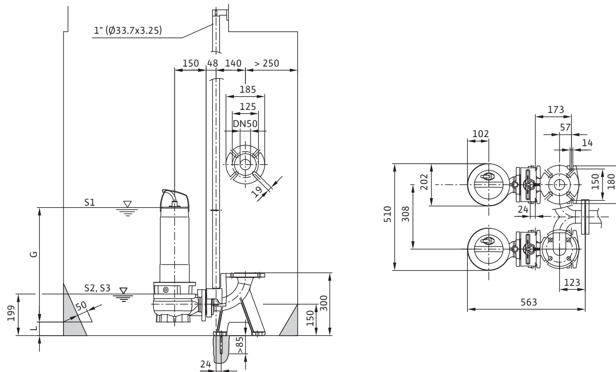
Габаритный чертеж Wilo-Rexa FIT V05 – стационарная погружная установка
