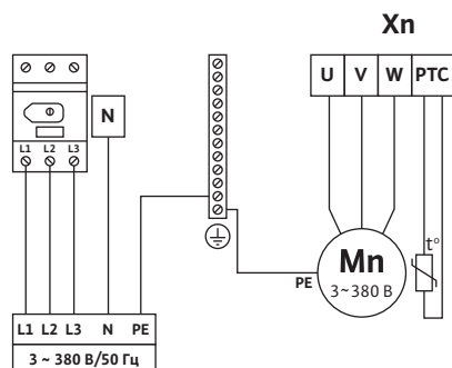
Схема подключения SK 712-d
