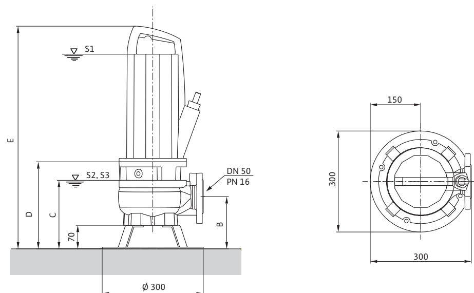
Габаритный чертеж Wilo-Rexa PRO V05 – мобильная погружная установка
