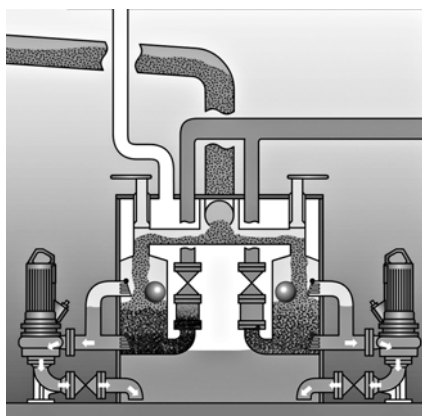
Процесс наполнения
