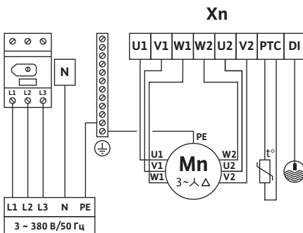
Схема подключения SK 712-sd
