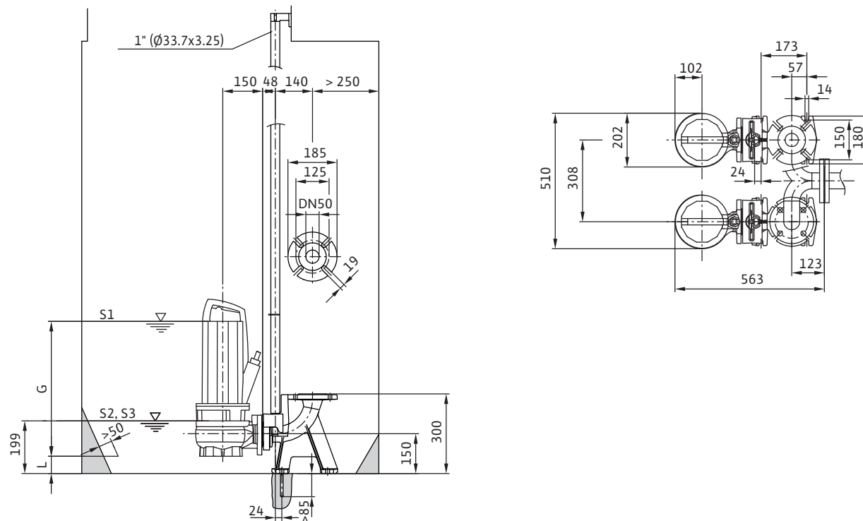
Габаритный чертеж Wilo-Rexa PRO V05 – стационарная погружная установка
