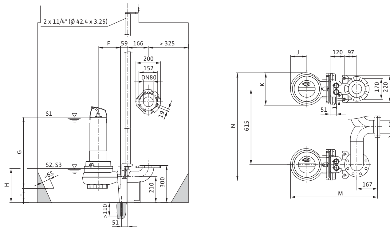
Габаритный чертеж Wilo-Rexa FIT V06 – стационарная погружная установка для DN 80
