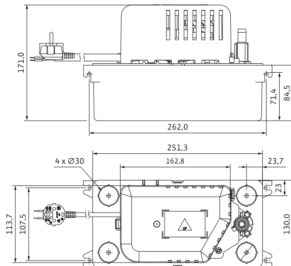
Wilo-DrainLift Con Plus
