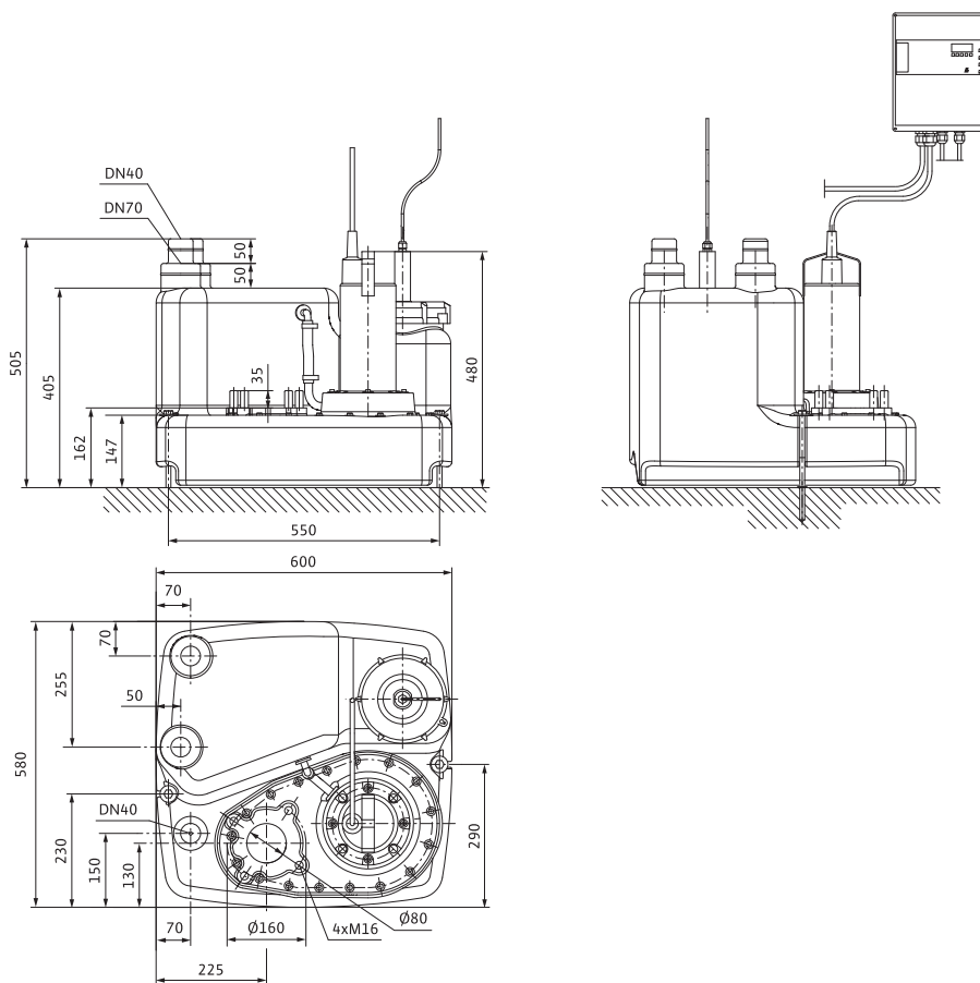
Габаритный чертеж
