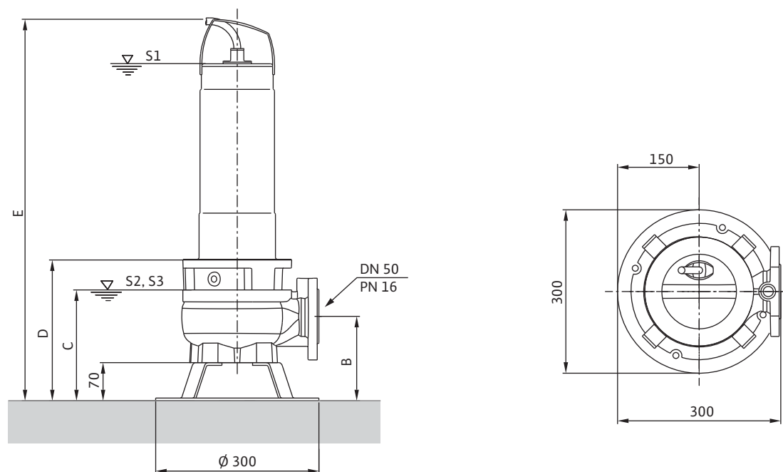
Габаритный чертеж Wilo-Rexa FIT V05 – мобильная погружная установка
