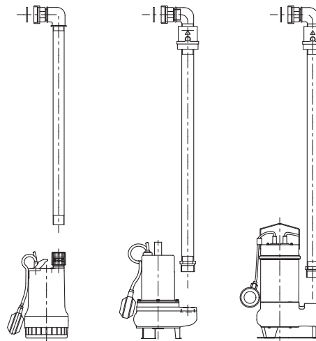
TMW 32/11
