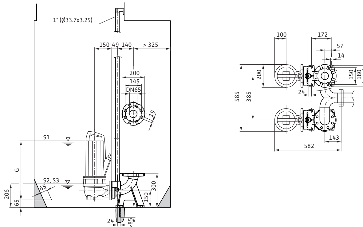
Габаритный чертеж Wilo-Rexa PRO V06 – стационарная погружная установка для DN 65
