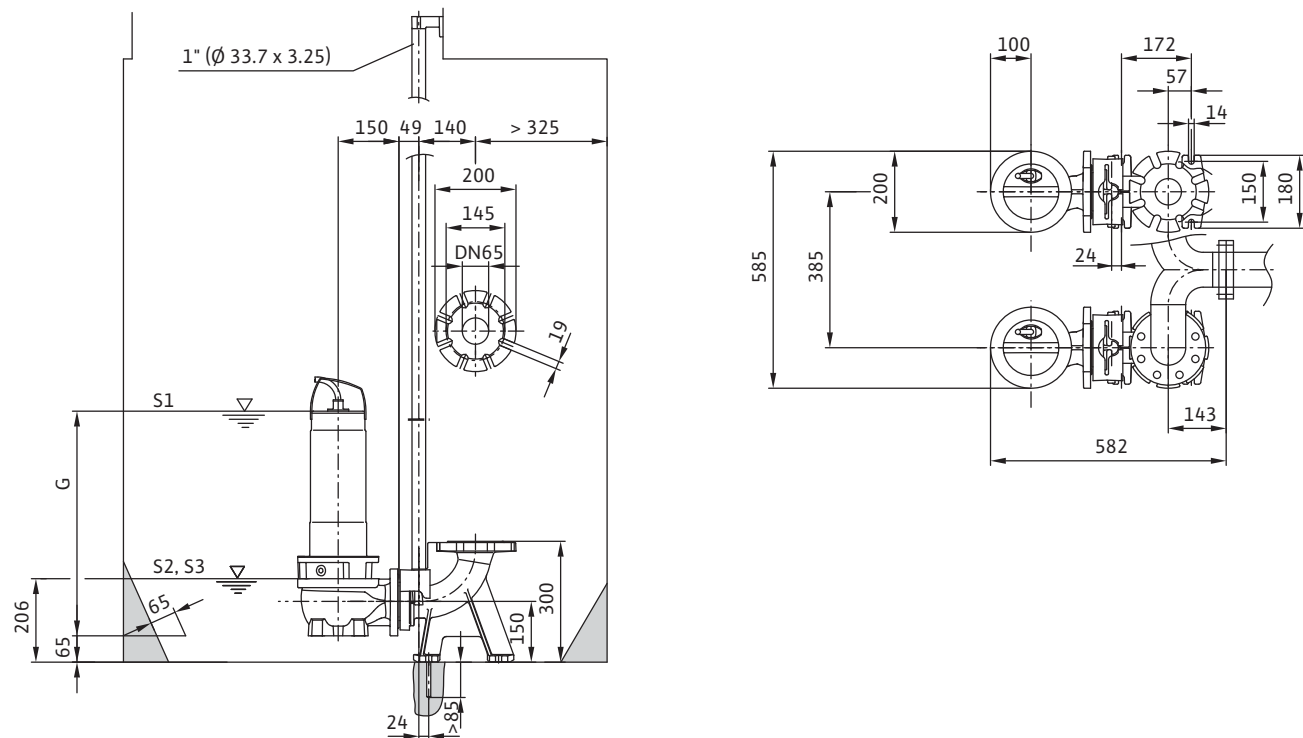
Габаритный чертеж Wilo-Rexa FIT V06 – стационарная погружная установка для DN 65
