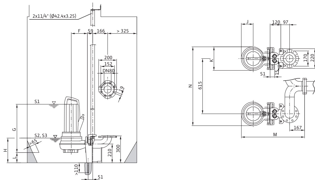
Габаритный чертеж Wilo-Rexa PRO V06 – стационарная погружная установка для DN 80
