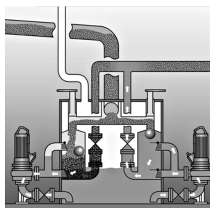
Слева: процесс заполнения. Справа: процесс перекачивания
