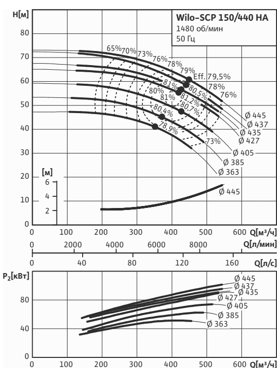
Wilо-SCP 150/440 HA
