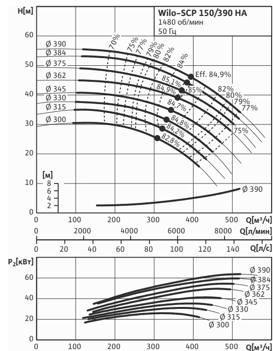
Wilо-SCP 150/390 HA
