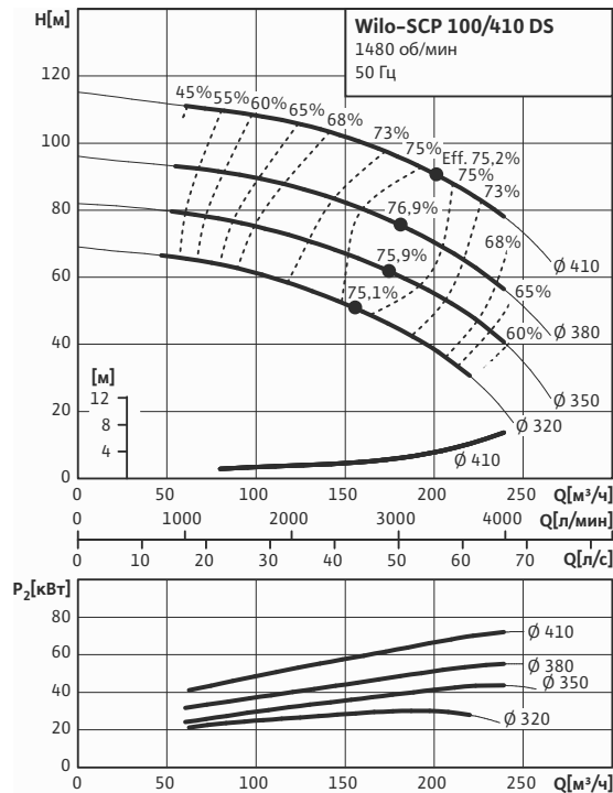
Wilо-SCP 100/410 DS
