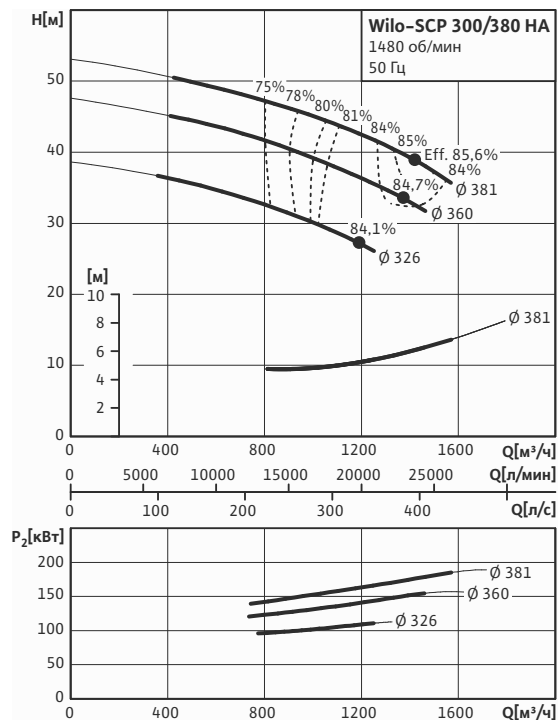
Wilo-SCP 300/380 HA
