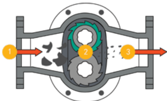
Измельчитель без фильтрующих барабанов
