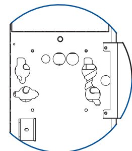
Вид В 2-х трубная система
