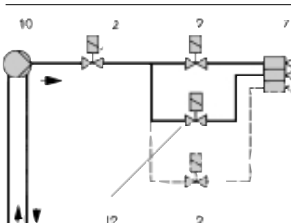
Комбинированные горелки GL 5 – 8 (ж/т часть двухступенчатая) GL 8 – 9 (ж/т часть трехступенчатая)
