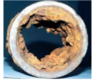
Рис. 2. Отложения в водопроводе питьевой воды
