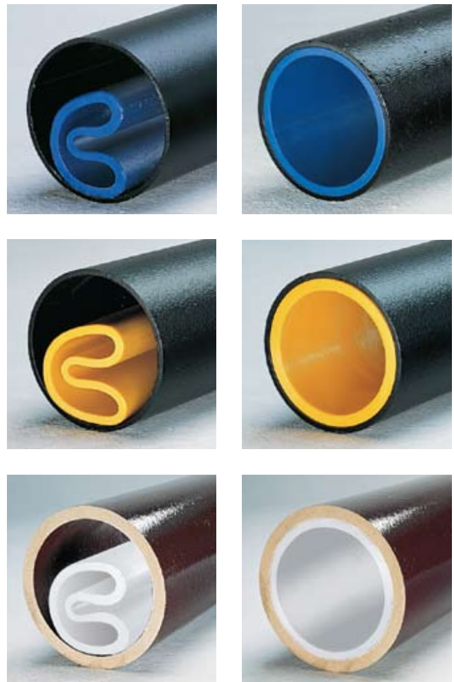
Рис. 21. Compact Pipe для обновления труб водопроводов, газопроводов и канализации
