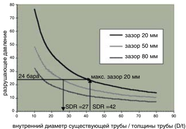
Рис. 47 Продолжительная (50 лет) способность перекрытия щелей для интерактивных труб из ПЭ 80.
