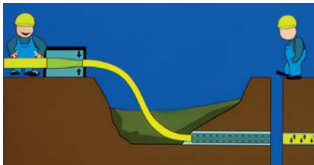
Рис. 11. Реконструкция плотноприлегающей трубой, формируемой на месте установки
