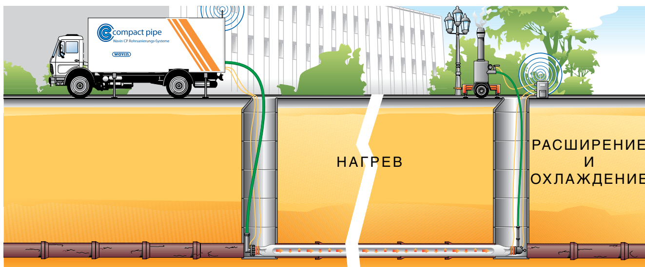
Рис. 27. Процесс установки Compact Pipe (продолжение)
