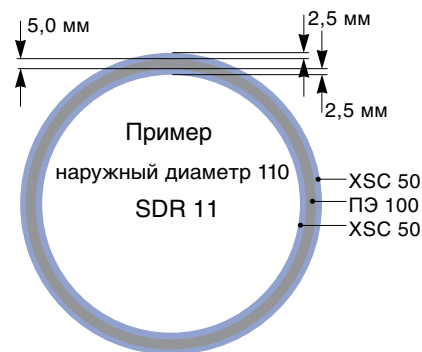
Рис. 41. Конструкция трубы Wavin TS
