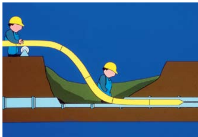
Рис. 9. Протяжка гибкой пластиковой трубы
