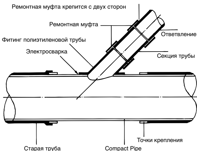
Рис. 31. Метод с раскапыванием для подсоединения ответвлений к канализационным трубам
