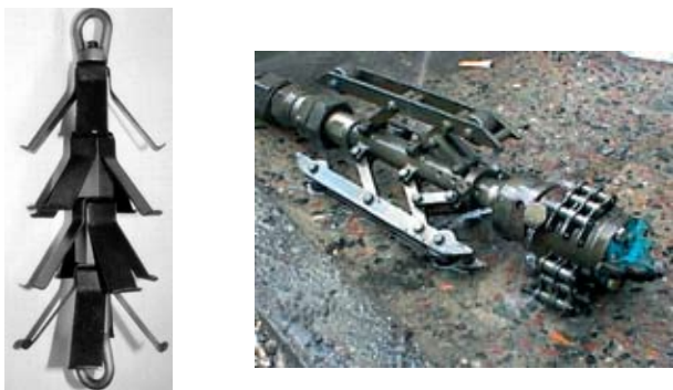
Рис. 7. Устройства для чистки – глубокий скребок (слева) и цепной скребок.
