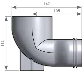
Горизонтальный переходник 90°
