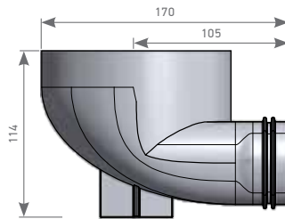
Горизонтальный переходник 90°
