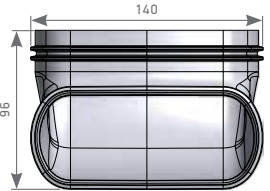
Вертикальный переходник 90°
