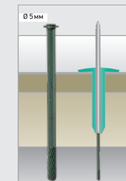
Крепление к бетону VILPE CROCO + KLA-дюбель
