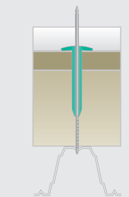
Крепление к металлу VILPE CROCO +KLA-шуруп
