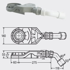
Гидрозатвор Advantix (плоская модель)
