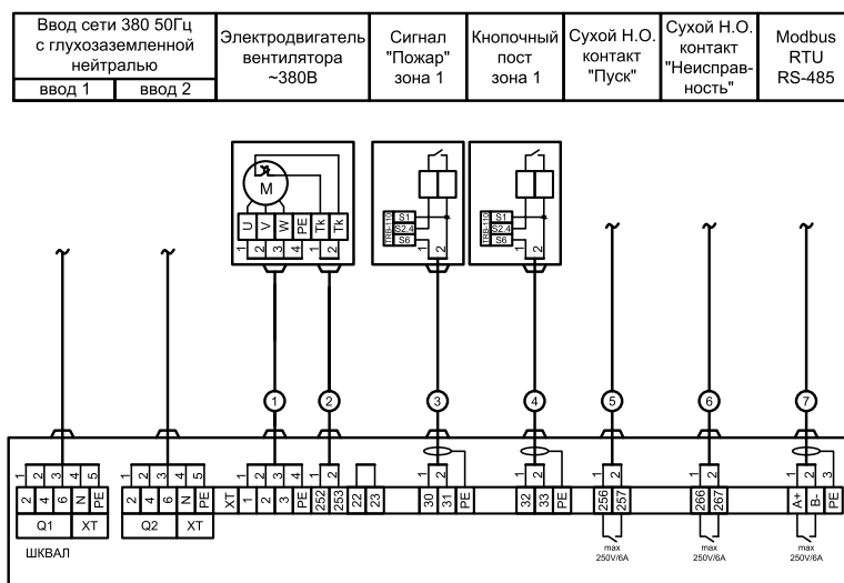
Схема 1 ШКВАЛ 110/210-ИР*1, ШКВАЛ 110/210-ИЧ*1
