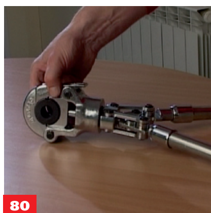
80 Поскольку обойма инструмента имеет шарнирное крепление к рукояткам, то рукоятки можно устанавливать в любое удобное положение
