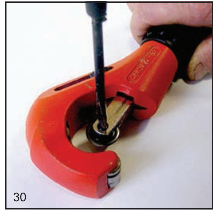
Если ролик роликового трубореза затупился или имеет заусенцы, производится его замена, для чего отверткой с плоским наконечником отвинчивается винт крепления ролика, ролик заменяется на новый и крепится винтом
