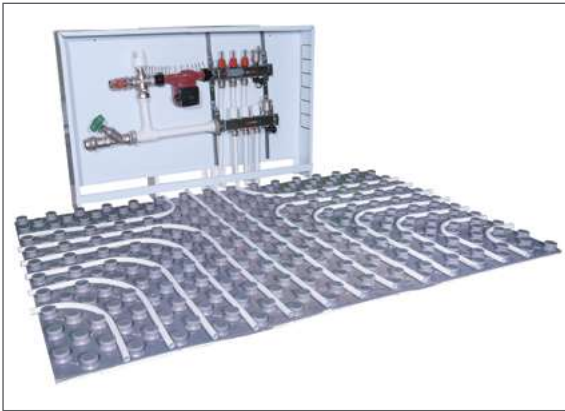
Схема комбинированного отопления помещений (водяной теплый пол и радиаторы). Площадь водяного теплого пола до 80 м 2 .
