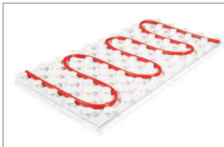
Плита без покрытия EasyFix 1000x500x40
