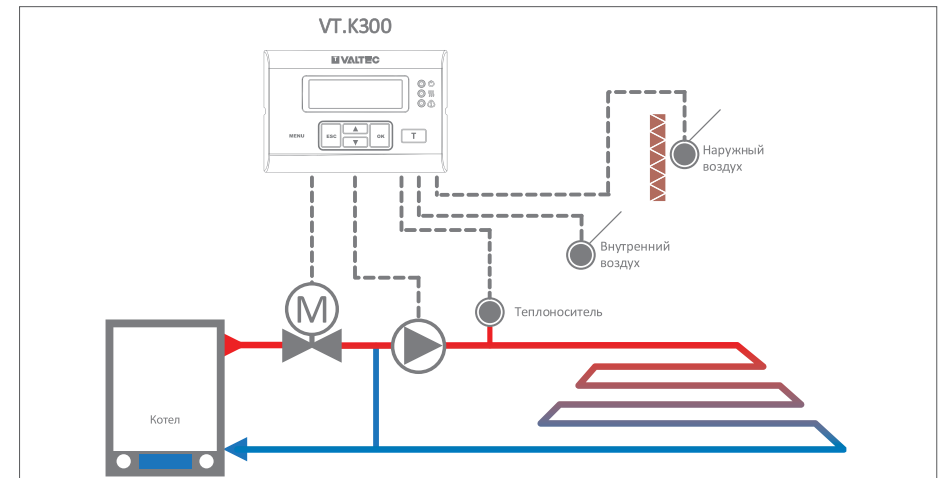
Рис. 24. Система управления теплым полом контроллером VT.K300
