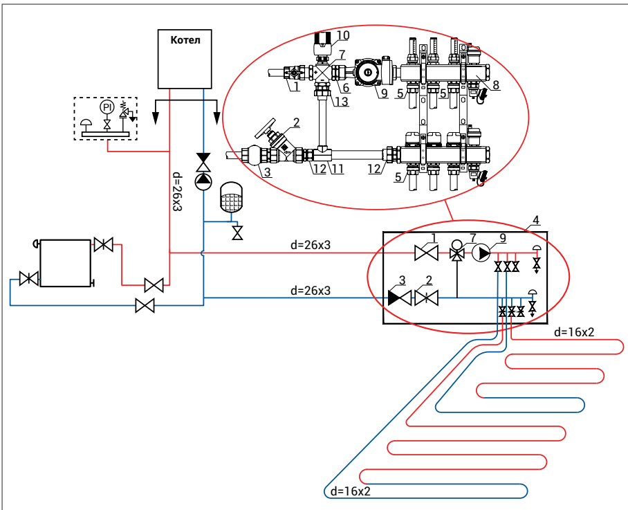
Схема комбинированного отопления помещений (водяной теплый пол и радиаторы). Площадь водяного теплого пола до 80 м 2 .
