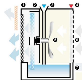
1) вариативный выпуск; 2) фильтрационный диск; 3) заполнение водой; 4) замена воздушного фильтра; 5) вентилятор; 6) всасываемый воздух; 7) рабочая поверхность
