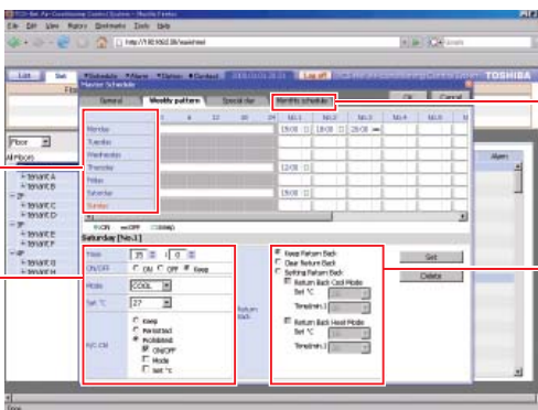
(экран компьютера)
