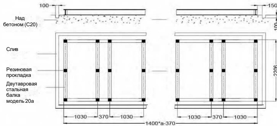
Чертеж двутаврового стального фундамента
