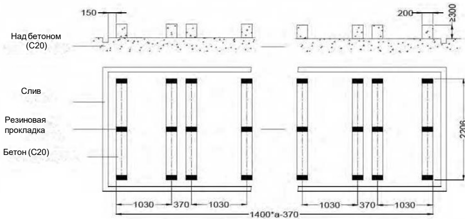
Чертеж бетонного фундамента
