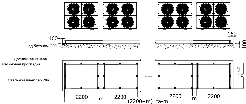
а) схема стального фундамента
