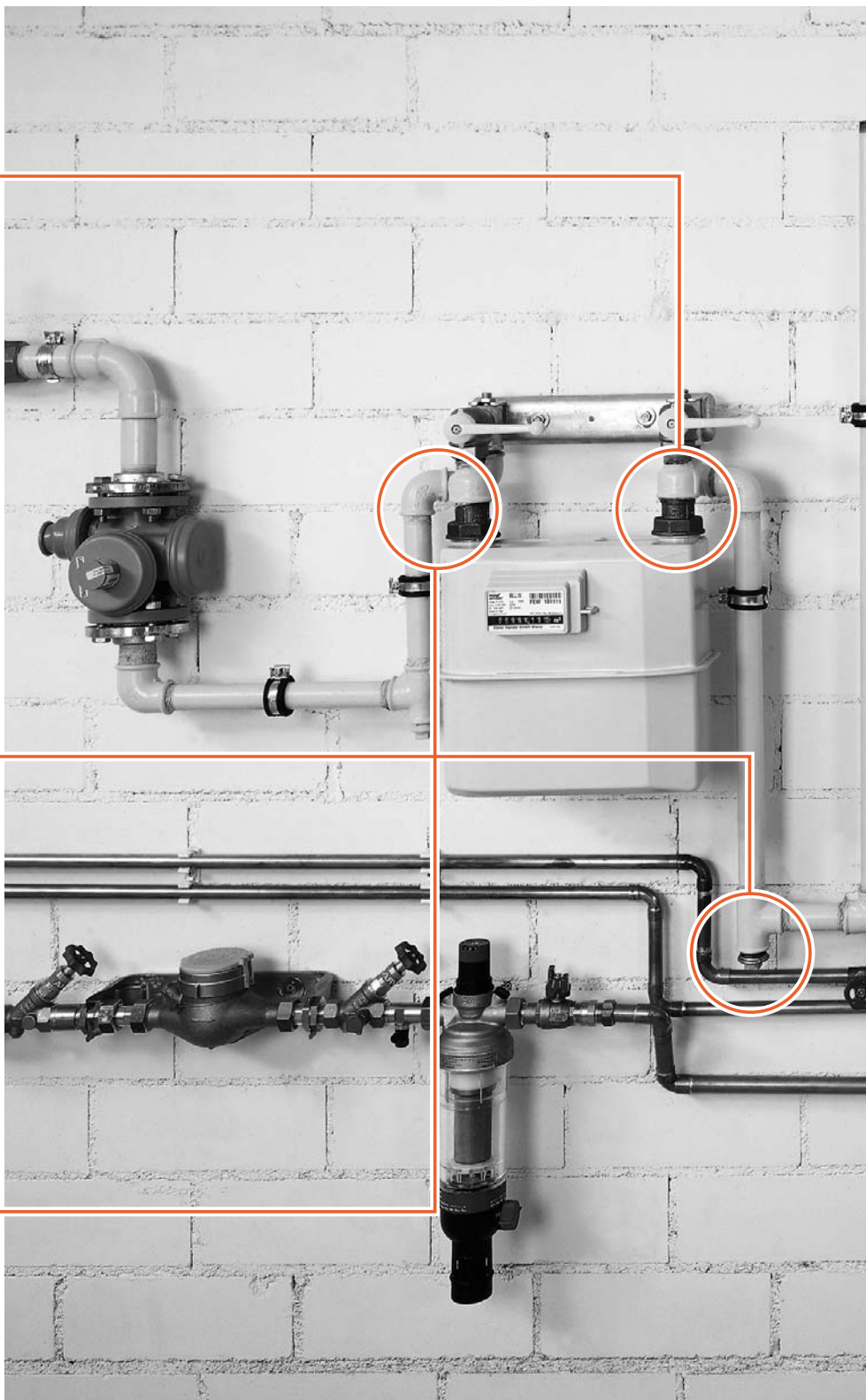
Проведение основных тестов с использованием прибора testo 312-2/3
