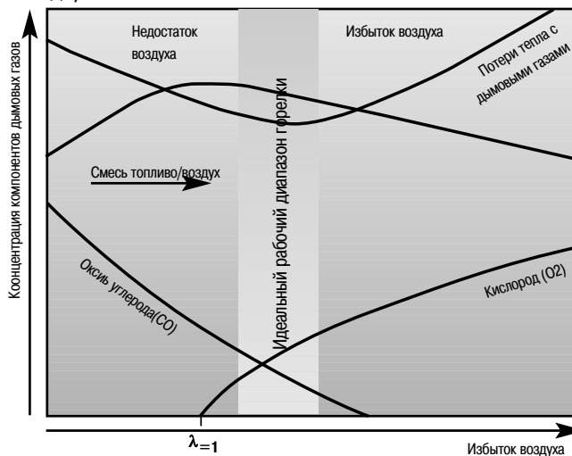
Рис. 10: Диаграмма процесса сгорания
