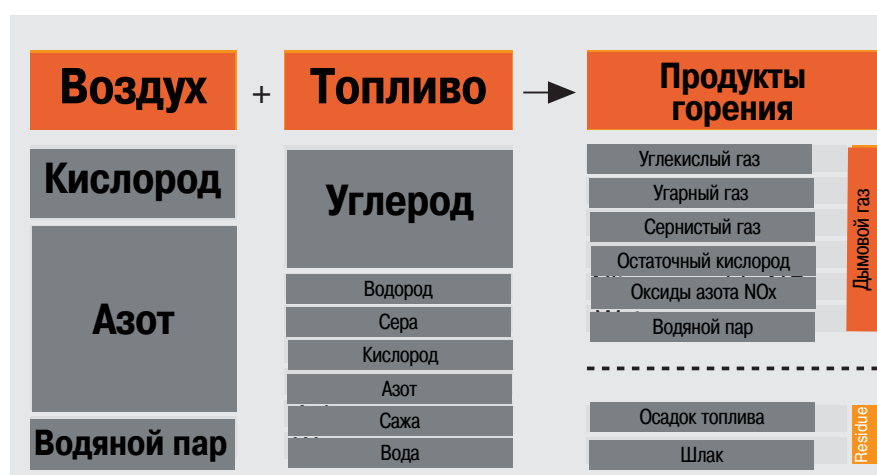
Рис. 2: Состав дымового газа
