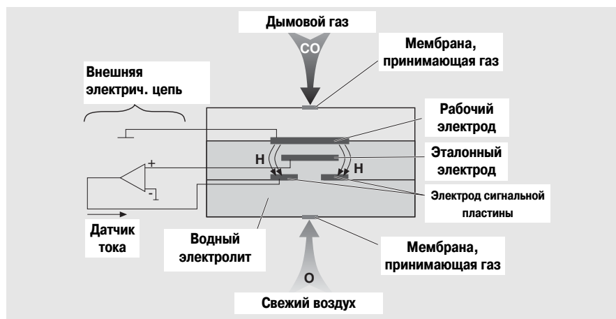
Рис. 28: Принцип работы сенсора CO
