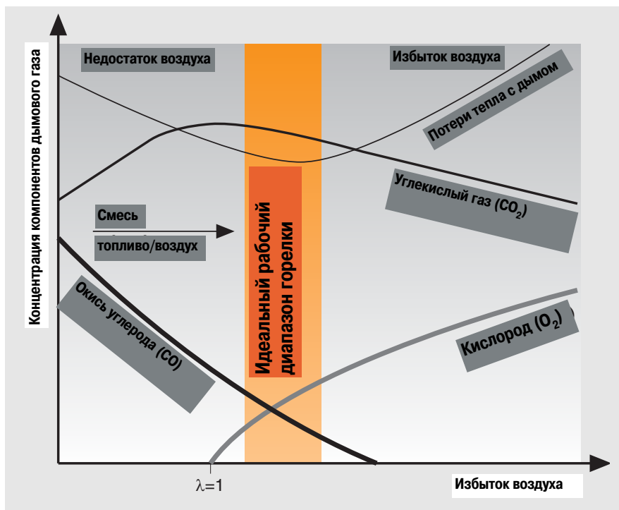
Рис. 23: Диаграмма процесса сгорания
