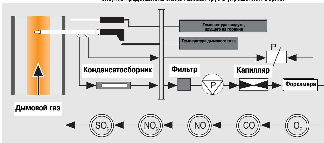
Рис. 31: Упрощённая схема газового тракта в анализаторе дымового газа
