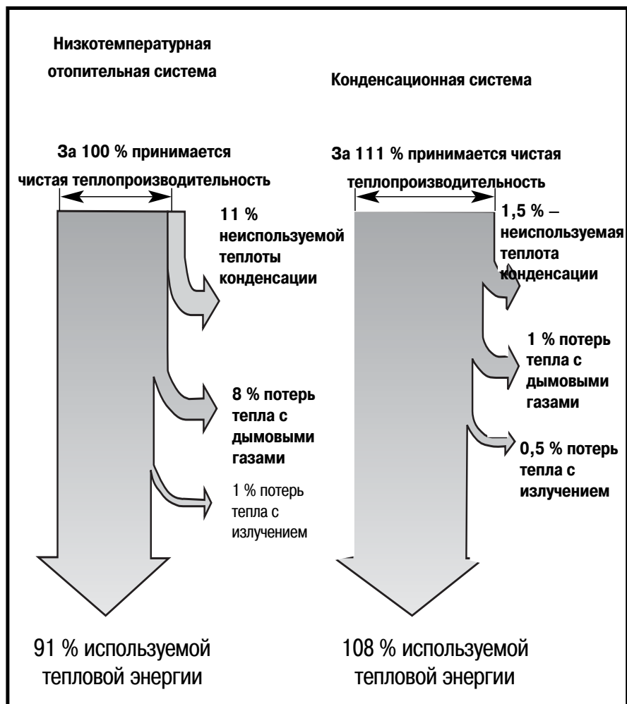
Рис. 17: Потеря энергии в низкотемпературных и конденсационных системах.
