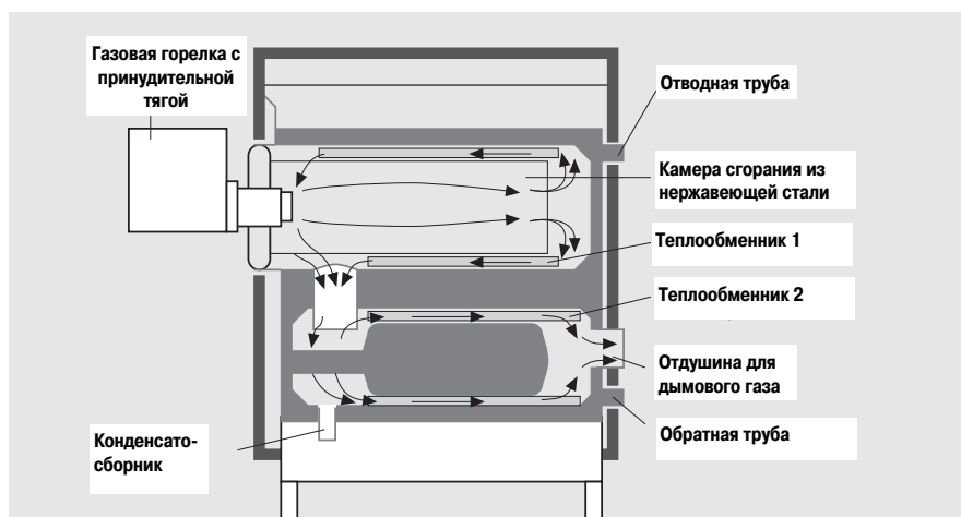
Рис. 8: Конструкция газового конденсационного котла
