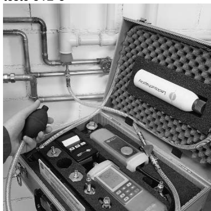
Проведение основных тестов с использованием прибора testo 312-2/3
