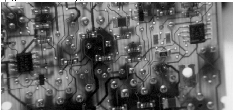
Рис. 30: Платы SMD на основе многоуровневой технологии
