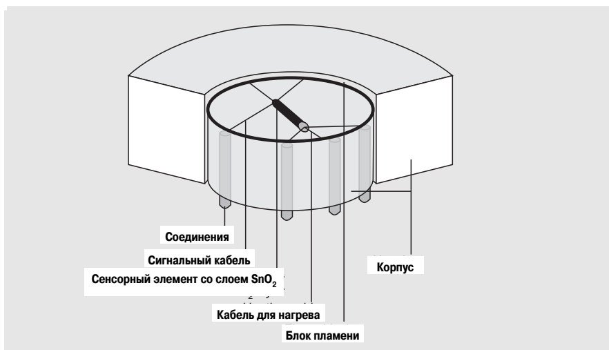
Рис. 29: Конструкция полупроводникового сенсора
