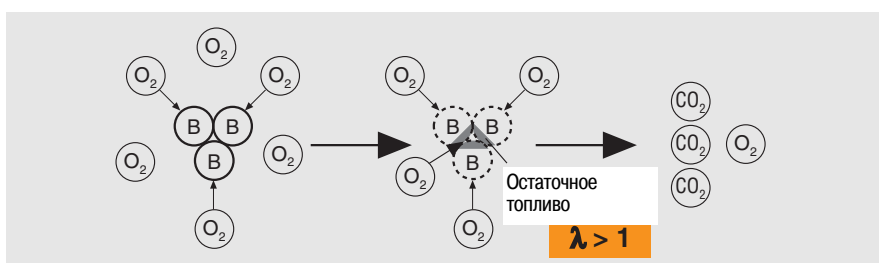
Рис. 4: Реальный процесс сгорания
