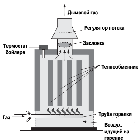
Рис. 7: Отопительная система с атмосферной горелкой
