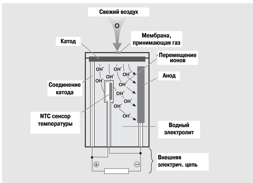
Рис. 27: Принцип работы сенсора O_2
