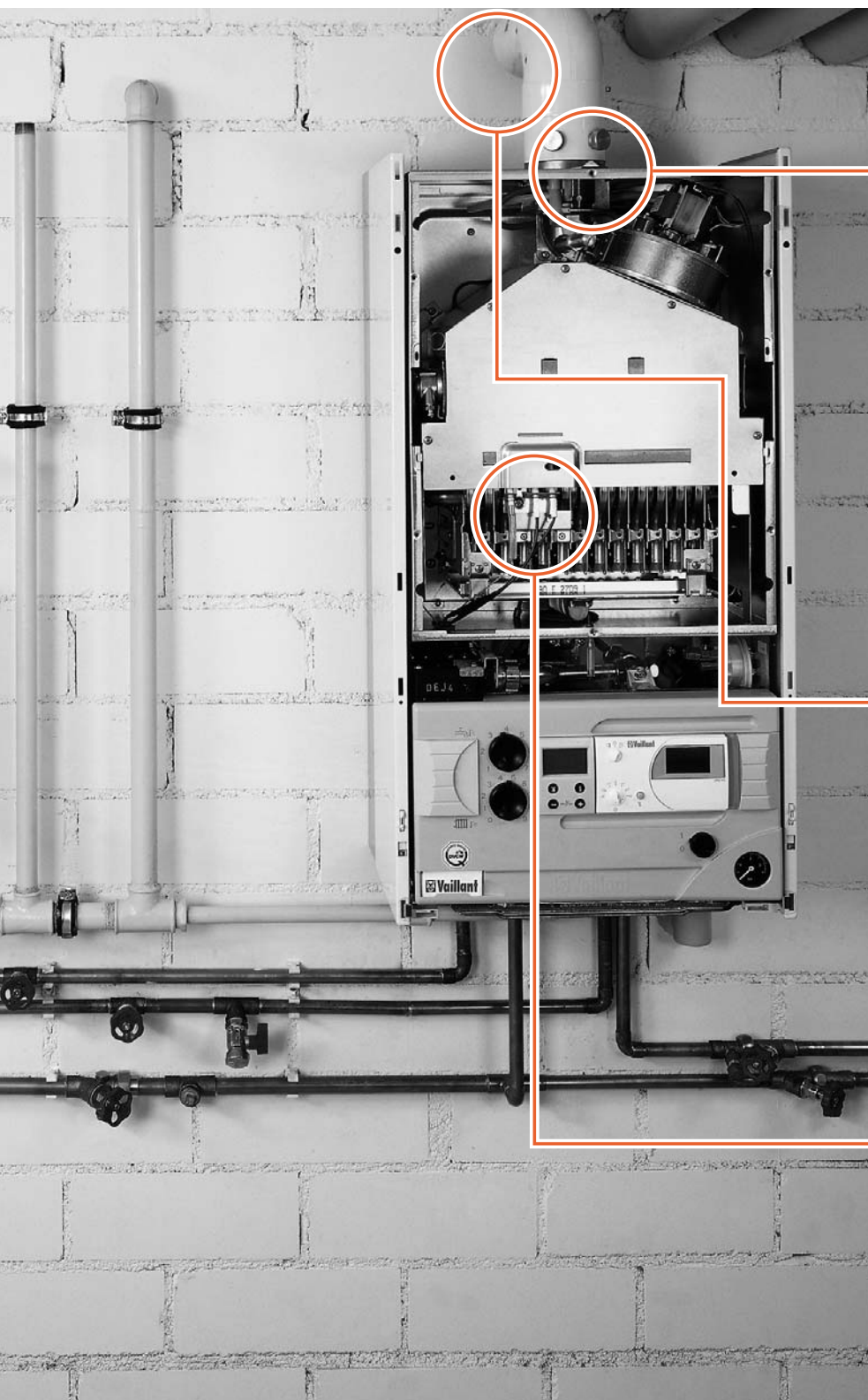
Тест дымовых газов с использованием приборов testo 327, 330-1LL, 330-2LL
