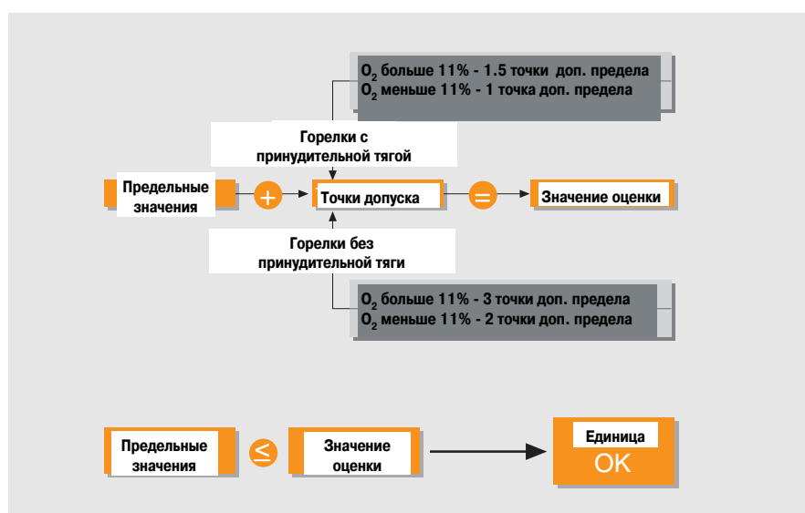
Рис. 14: Диаграмма расчёта оценочного значения
