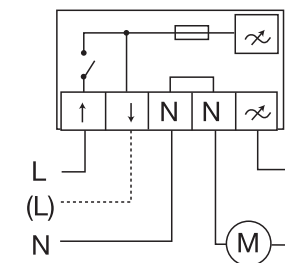
Фазный проводник L, указанный сплошной линией, оснащен устройством размыкания цепи питания вентилятора.
