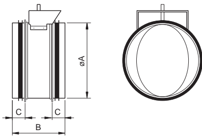
EFD 160-315
