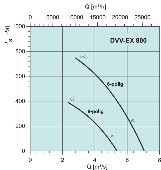
DVV-EX 800D6
