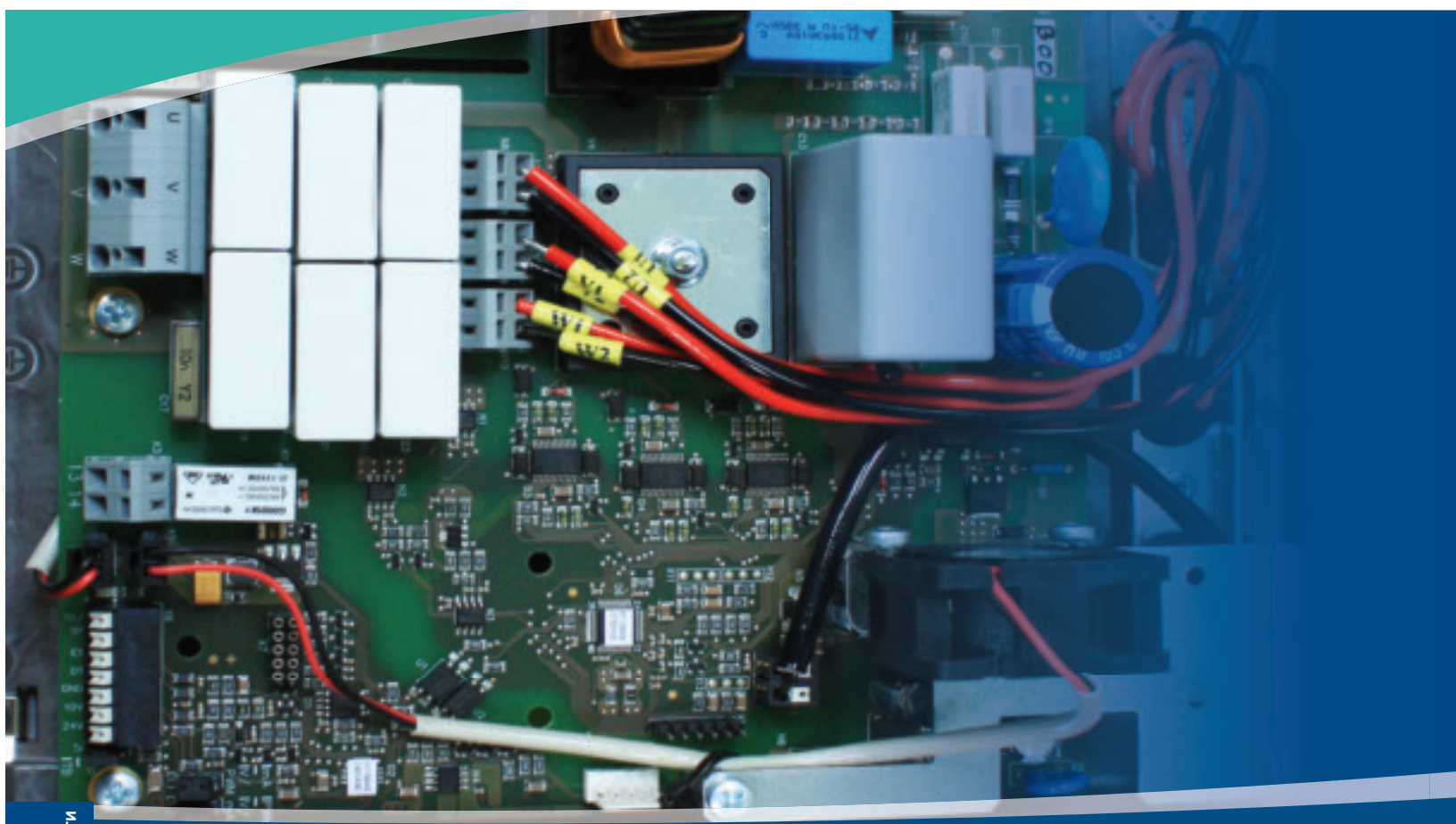
Регулятор скорости, трансформаторы
