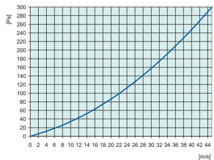
LRK (F) Аэродинамическое сопротивление
