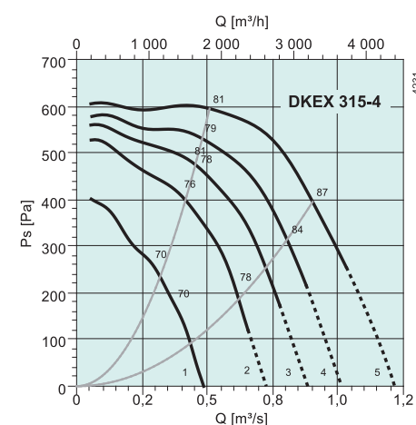
Мин. статическое давление 250 Па
