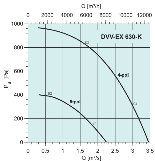
DVV-EX 630D4-K
