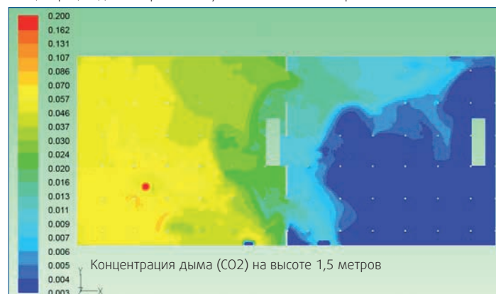
Концентрация дыма через 5 минут после начала пожара
