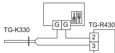
Схема подключений при использовании функции уменьшения температуры ночью
