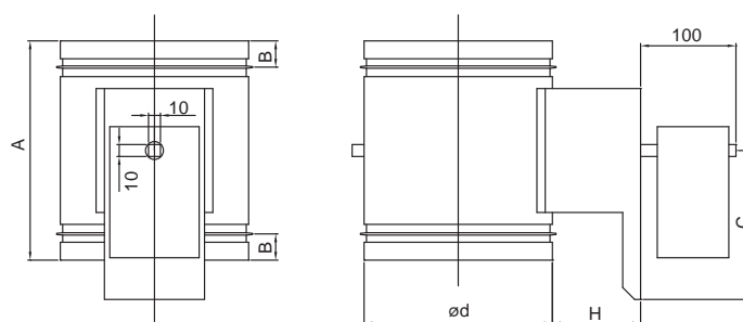
EFD 400-630
