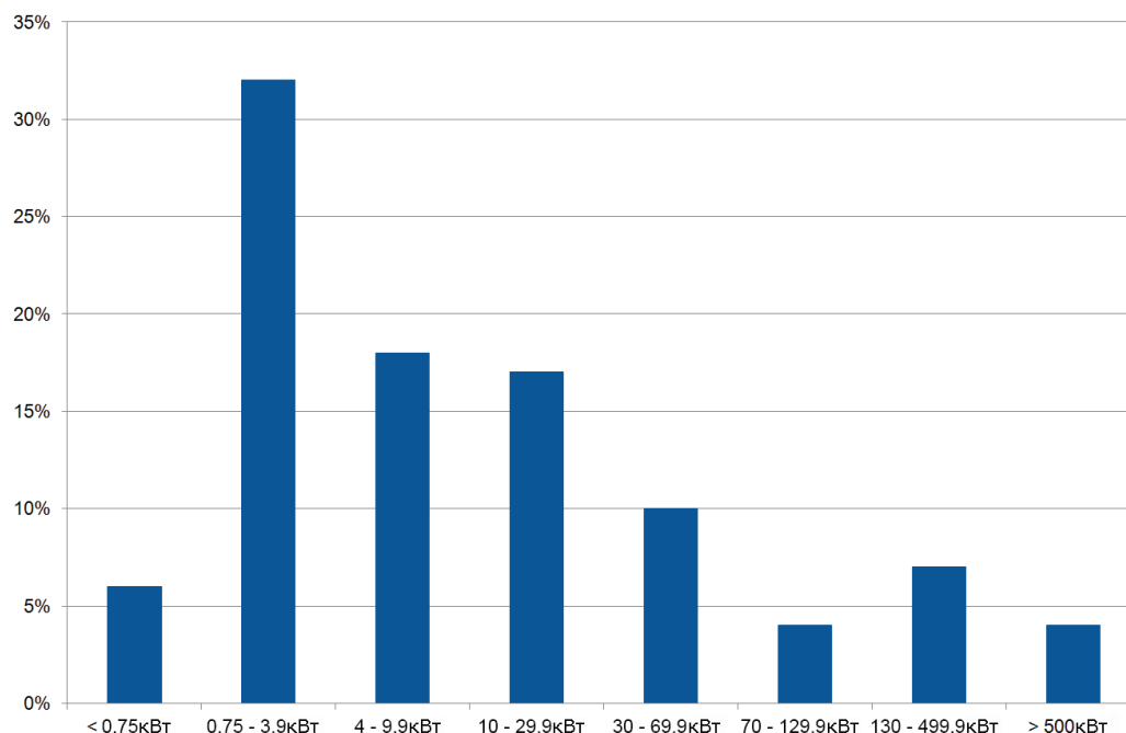
Электродвигатели по группам номинальной мощности и их доля от мирового электропотребления
