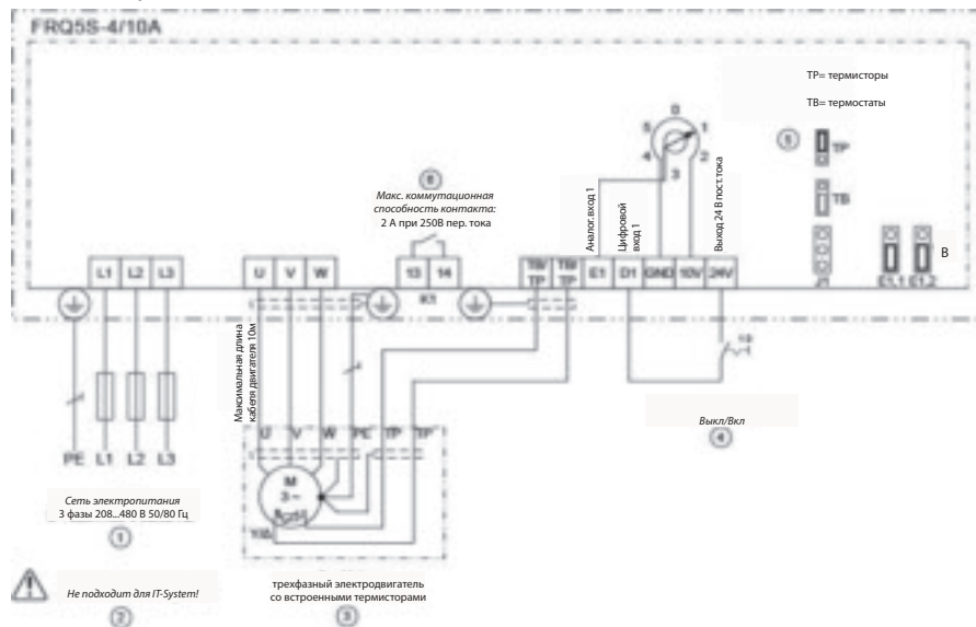
Схема электрических подключений FRQS 4/10A
