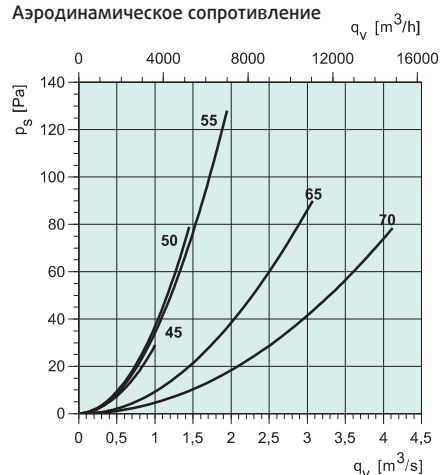
Аэродинамическое сопротивление
