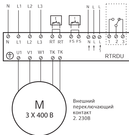
Фазный проводник L, указанный сплошной линией, оснащен устройством размыкания цепи питания вентилятора.
