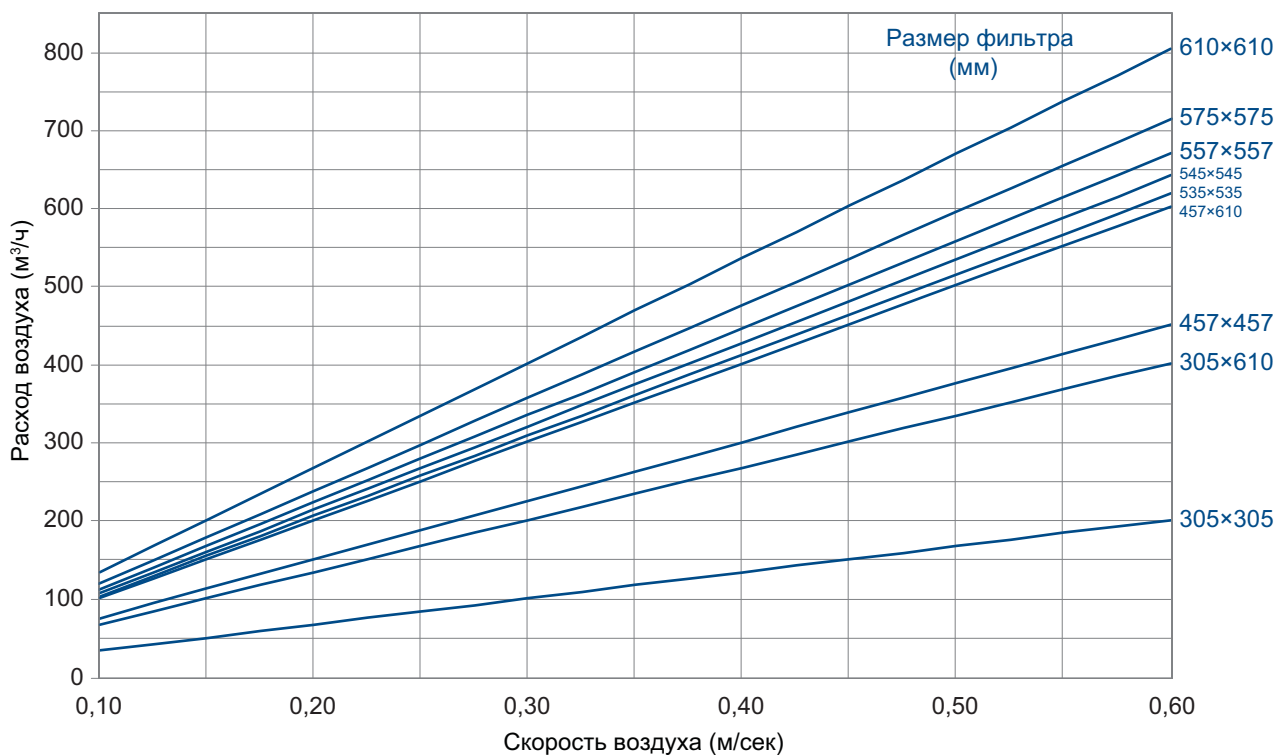
Диаграмма 2. Зависимость между фронтальной скоростью воздуха и расходом воздуха на корпусе CFC без лицевой панели, в комплекте с фильтром Н14, толщиной 80 мм (уплотнение из неопрена или гелевым уплотнением).
