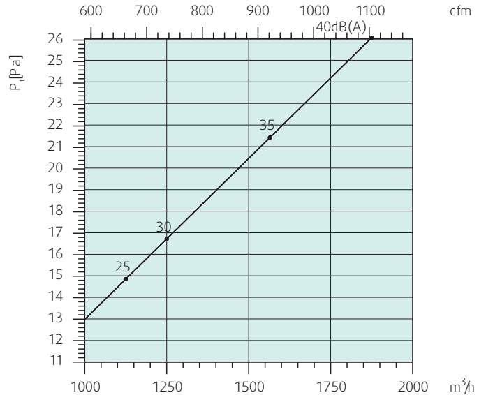
TSD-630 Режим отопления (вертикальная подача воздуха)
