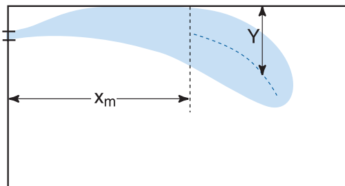
Рис. 13. Точка отрыва воздушной струи ( x_m ) и отклонение ( \gamma )
