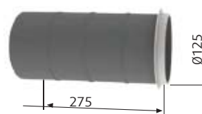
Проходной патрубок
