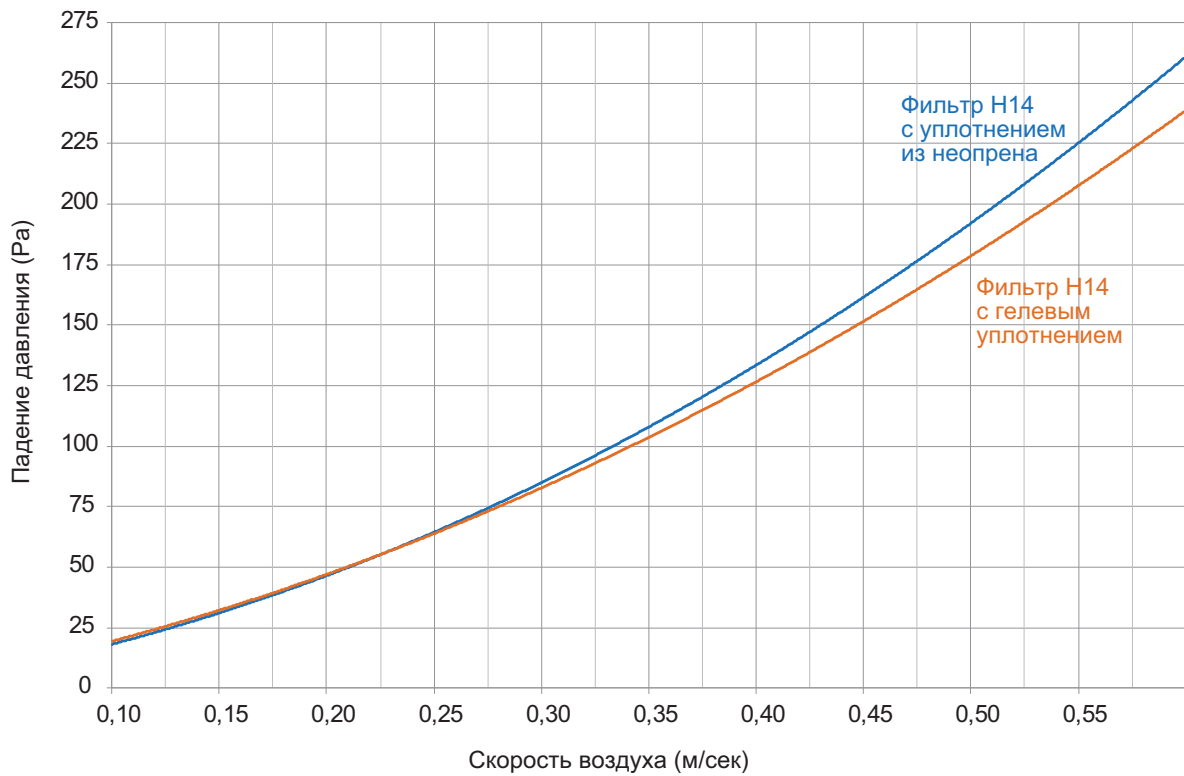
Диаграмма 1. Зависимость между фронтальной скоростью воздуха и падением давления на корпусе CFC без лицевой панели, в комплекте с фильтром Н14, толщиной 80 мм (уплотнение из неопрена или гелевым уплотнением).
