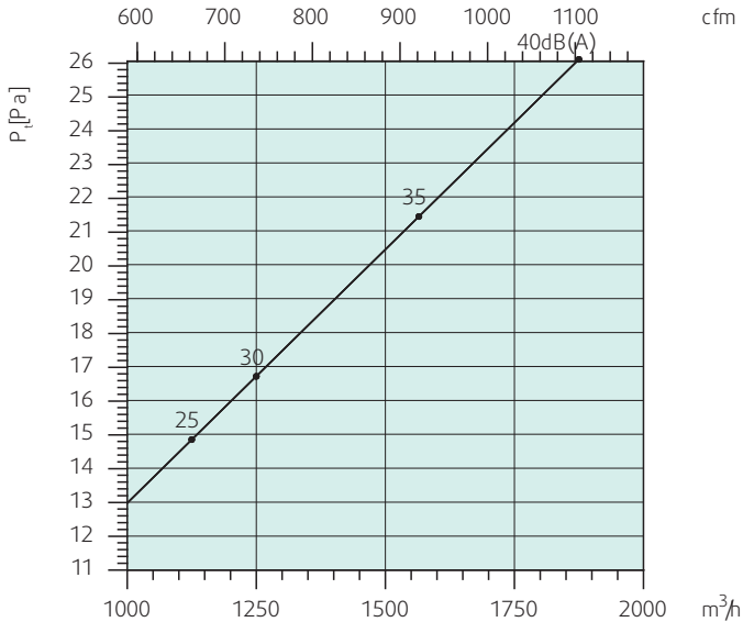
TSD - 630 Режим охлаждения (горизонтальная подача воздуха)
