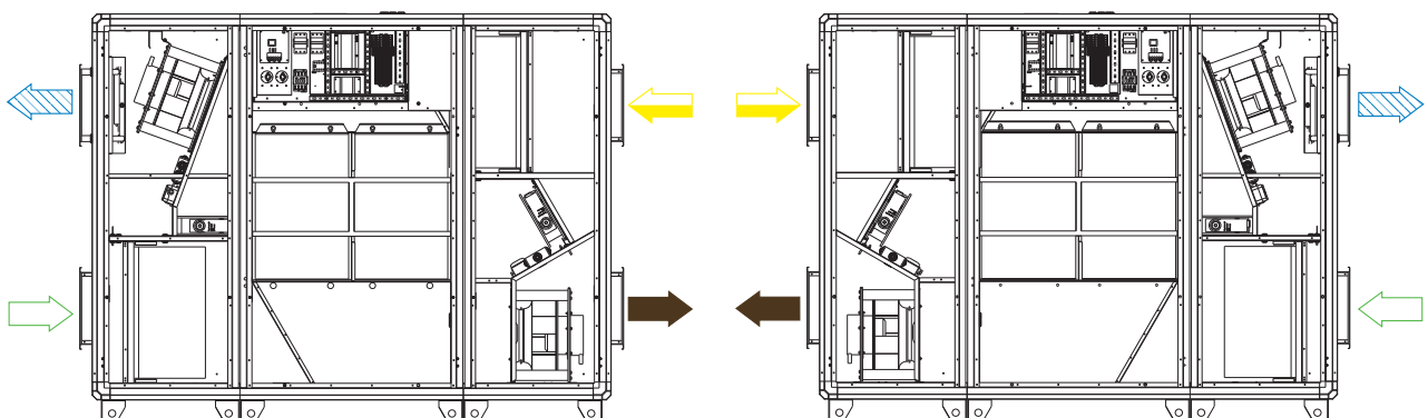
Левосторонний агрегат
