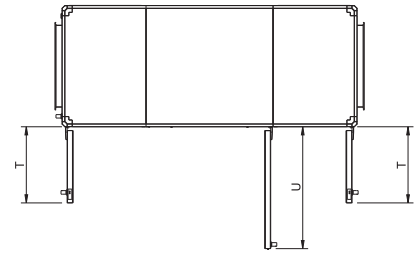
Вид сверху. Левосторонний агрегат
