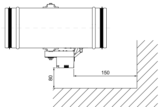
Установка Optim-R-BLC. Минимальное расстояние до стены
