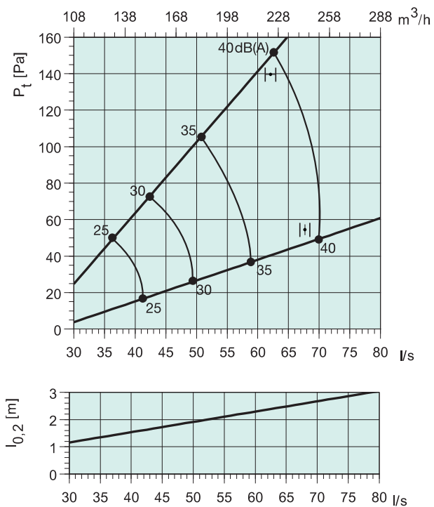
TSK 160 + THOR 125-160
