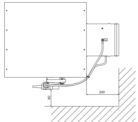
Установка Optim-RS-BLC. Минимальное расстояние до стены
