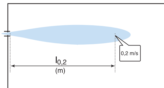
Рис. 14. Понятие "Длина струи"
