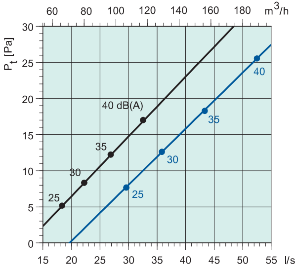
Sinus-DC/DR-1501
