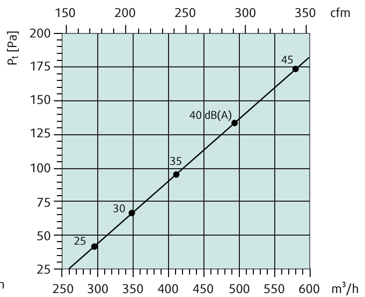
AJD 200
