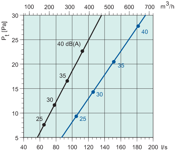
Sinus-DC/DR-1503
