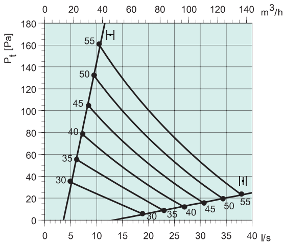
SPI-80
