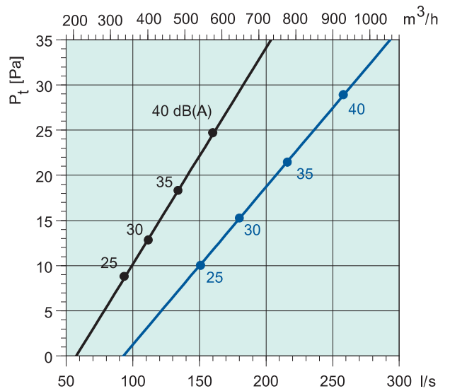
Sinus-DC/DR-1504
