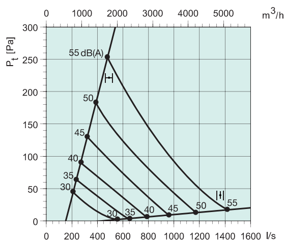
SPI-400
