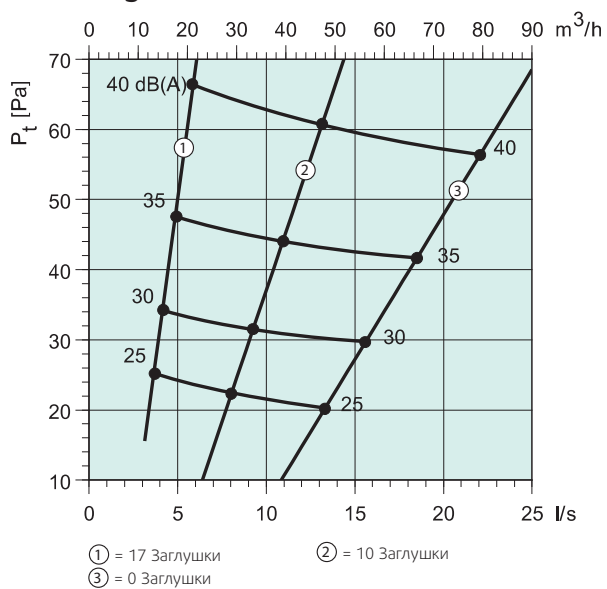
Elegant VT 100
