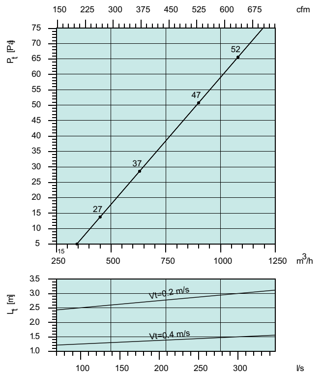
VVKR - 625-32
