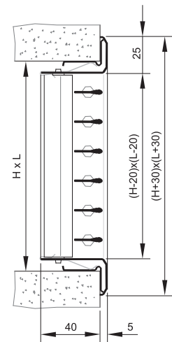
NOVA-A-2
