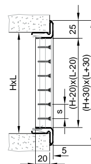
NOVA-L-1-2-LxH
