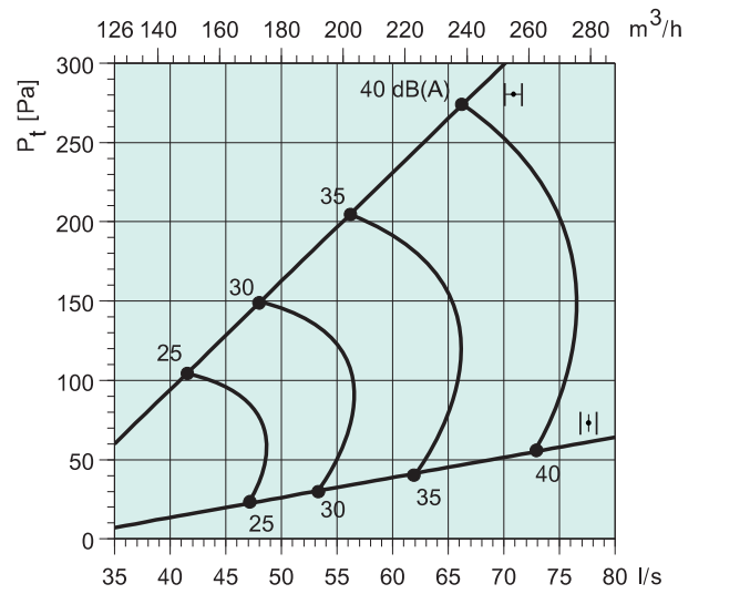
Sinus-A 200-L + THOR 160
