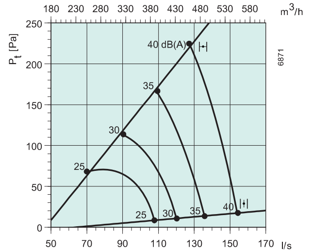
Боковой зазор открыт
