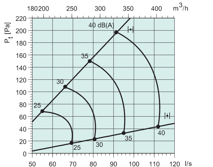
Sinus-A 250-L + THOR 200
