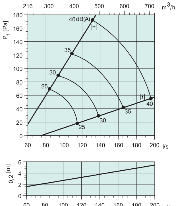
TSK 315 + THOR 250-315
