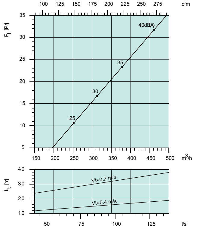
VVKR - 500-24
