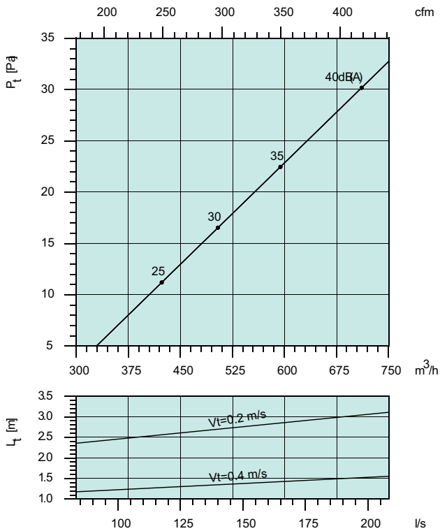
VVKR - 600-32
