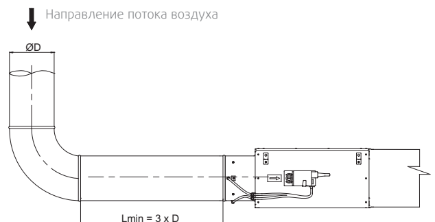
Установка Optim-RS-BLC. Минимальное расстояние до стены
