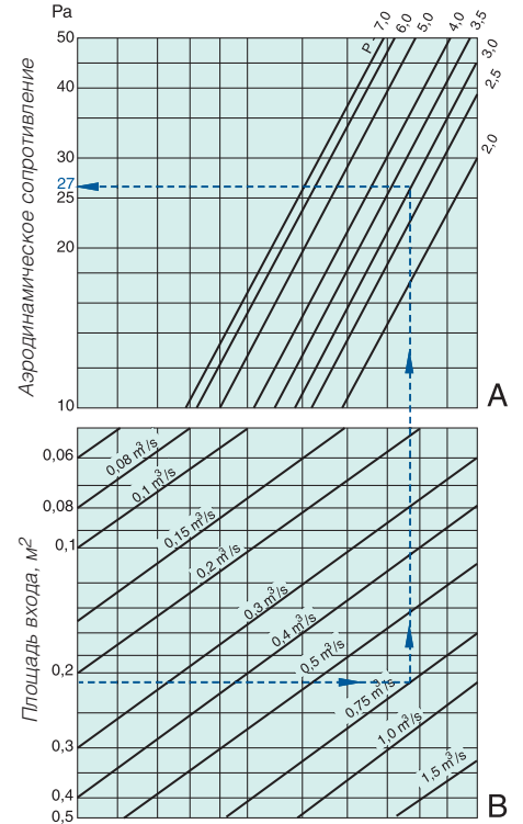
График расчета падения давления в шумоглушителе LDR
