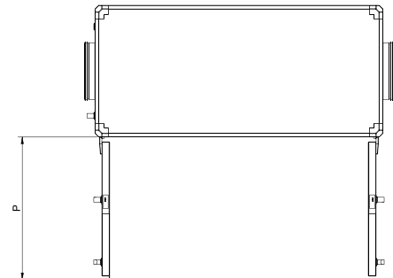
Вид сверху. Левосторонний агрегат
