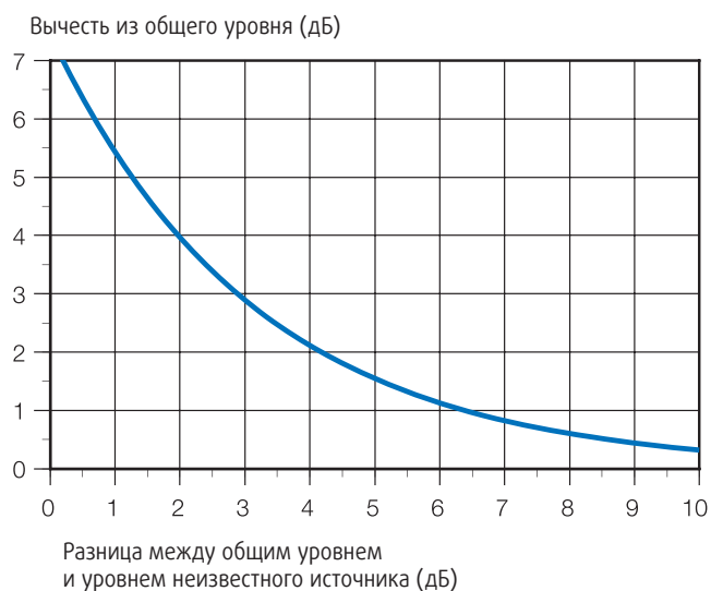
Рис. 6. Логарифмическое вычитание
