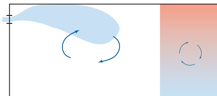
Рис. 16. Вторичные вихри образуются в самом дальнем конце помещения, куда не доходит воздушная струя
