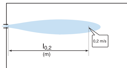
Рис. 14. Понятие "Длина струи"
