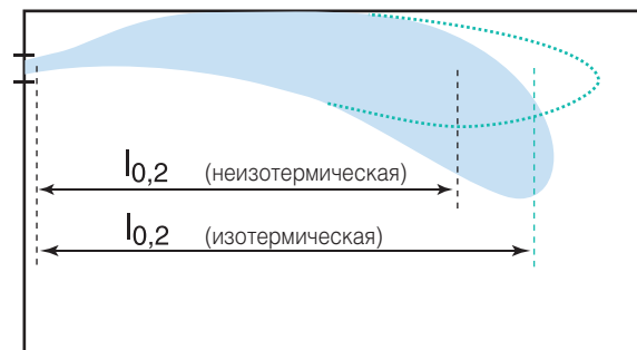
Рис. 23. Разница между длиной изотермической и неизотермической струй.
