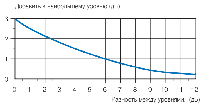
Рис. 5. Логарифмическое сложение
