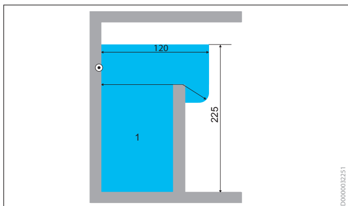
Вид сбоку со стационарной перегородкой и неперекрывающий радиус
